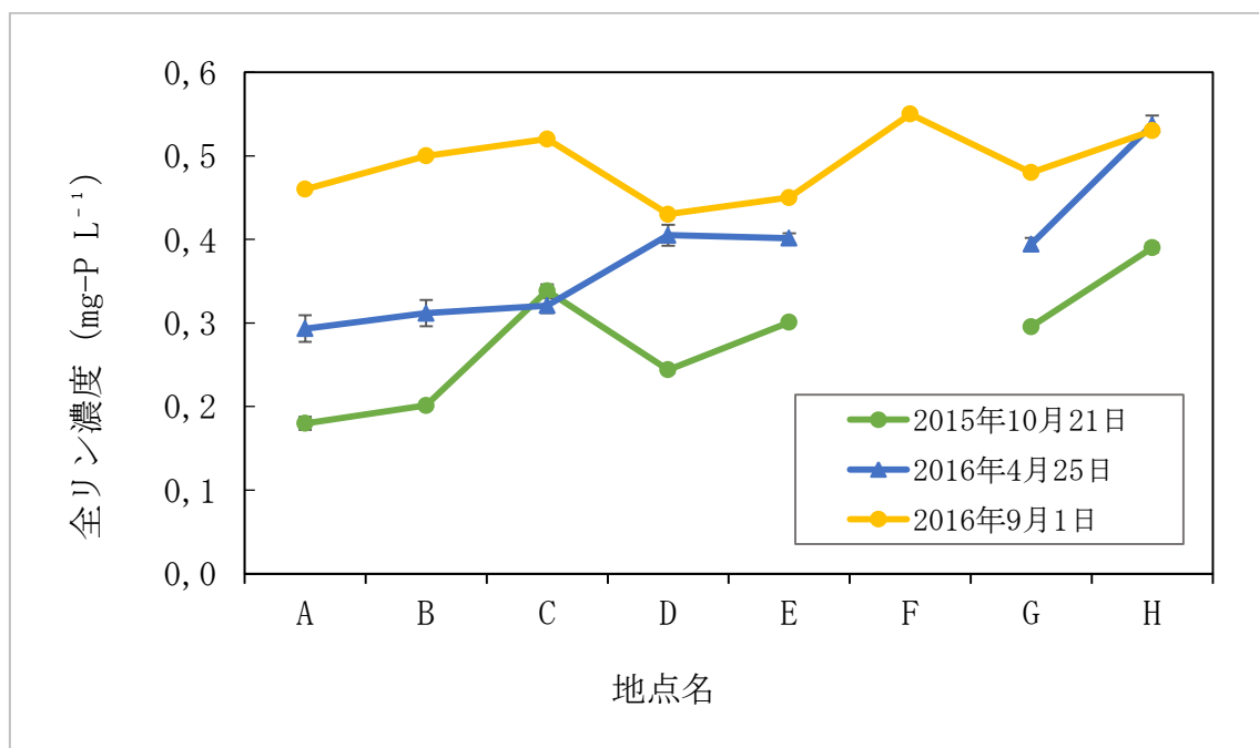
図 5 : 半尾川の全リンの上流から下流への変化
