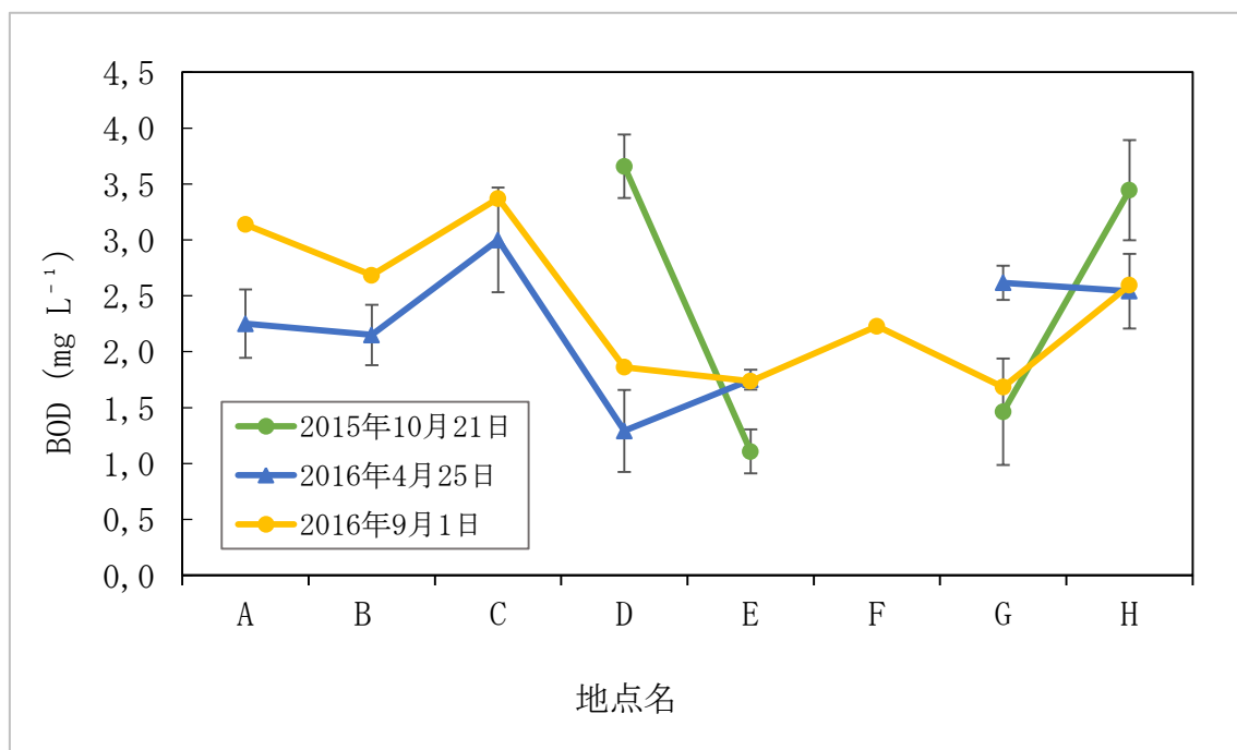
図 3 : 半尾川の BOD の上流から下流への変化
