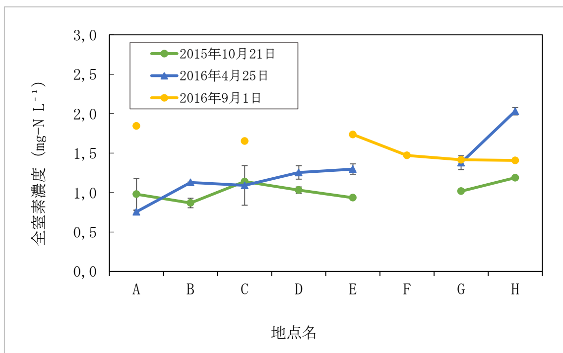
図 4：半尾川の全窒素の上流から下流への変化
