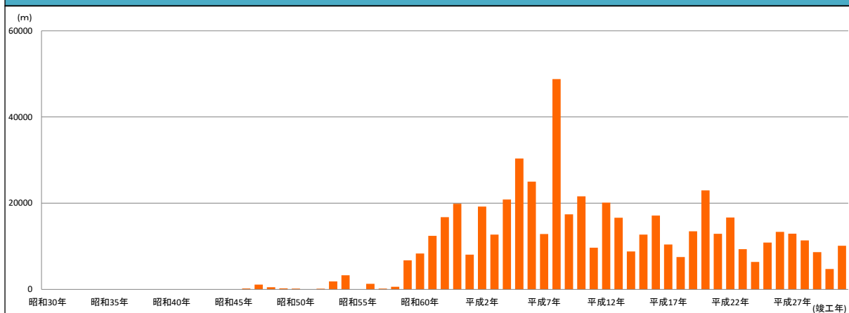
下水道（管）の竣工年別の分布状況（延長）
