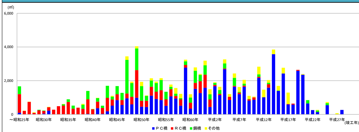
橋りょうの竣工年別の分布状況（面積）
