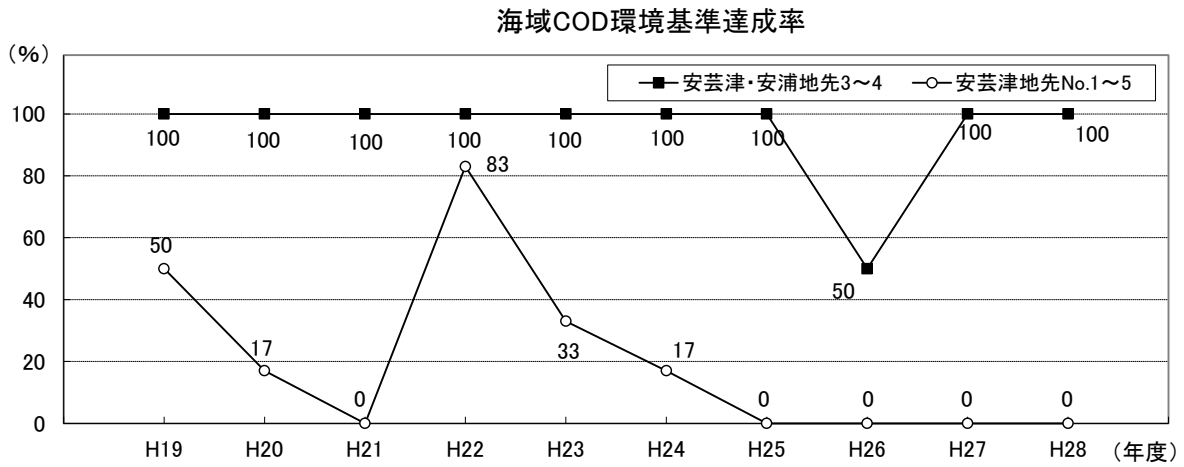
海域のCOD測定結果（平成28年度）
