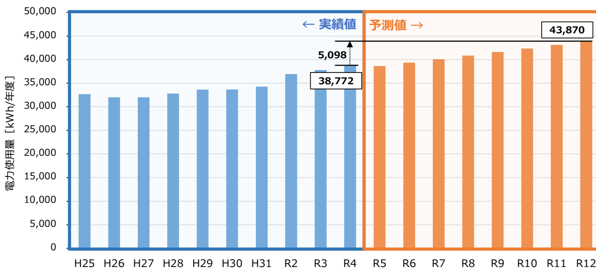
図 4-6 市有施設の使用電力量の実績と将来の見込み
