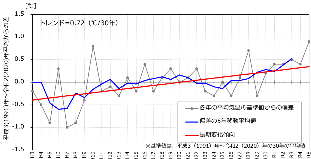
図 1-6 平均気温偏差の状況
