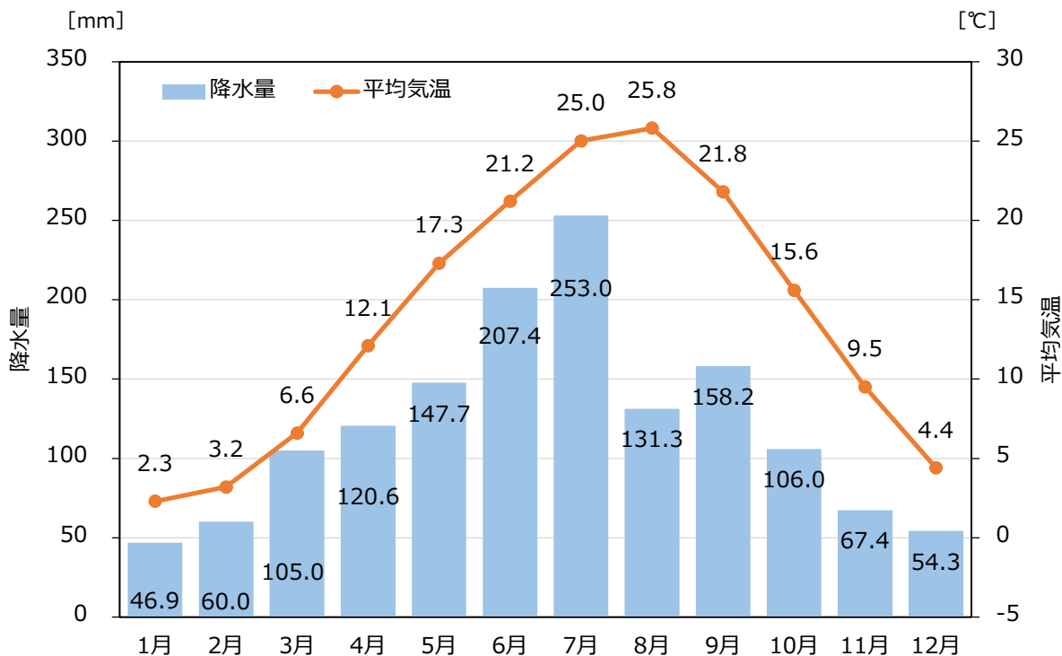
図 1-7 平均気温・降水量（平成 3（1991）年～令和 2（2020）年）
