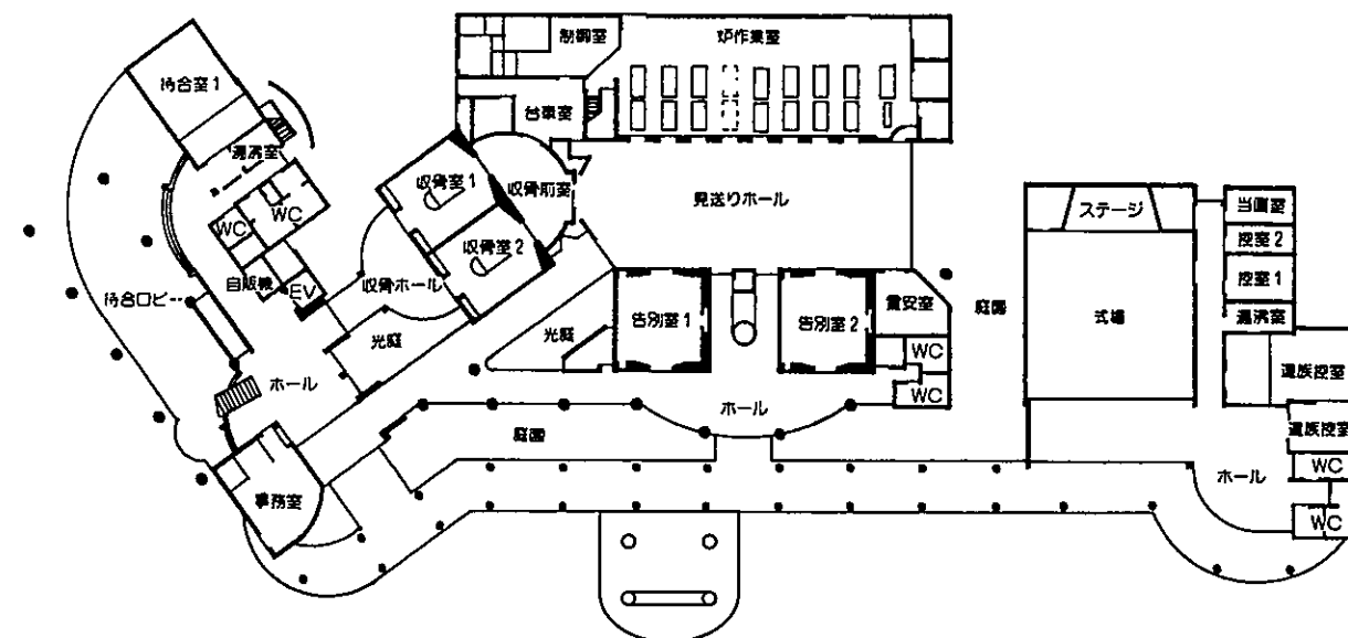
1 階平面図
