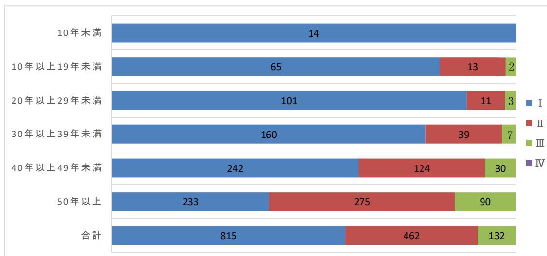
図 3-6 建設経過年数と定期点検結果に基づく健全性の診断区分（未点検橋梁 28 橋を除く）
