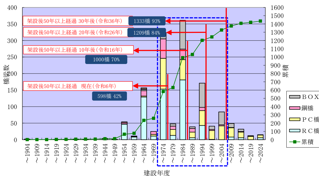
図 3-3 橋梁架橋年度別数
