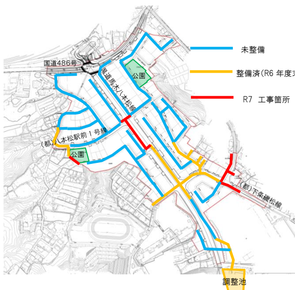
雨水管渠平面図
