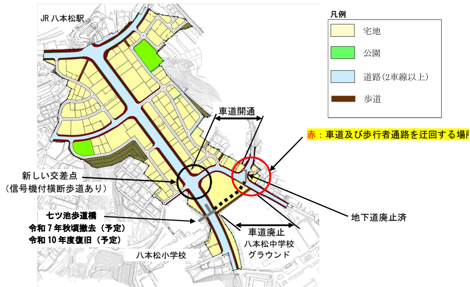
計画平面図(イメージ)
