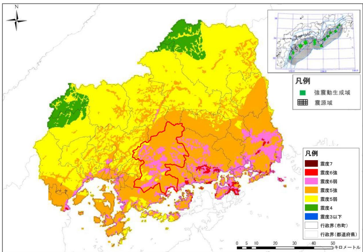
図 7-2 地震の震度分布（南海トラフ巨大地震（陸側ケース）
