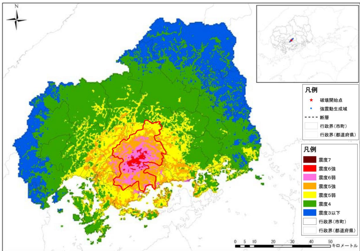
図 7-1 地震の震度分布（東広島市直下地震）
