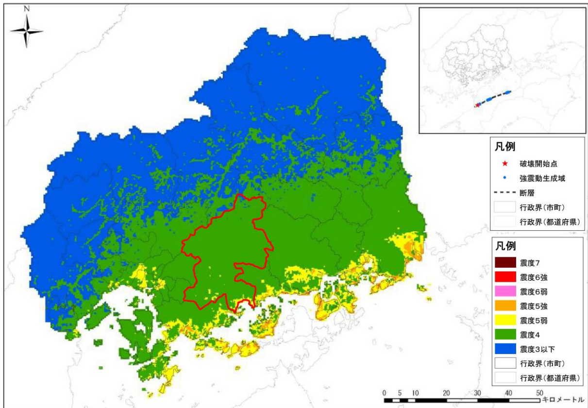
図 7-5 地震の震度分布（石鎚山脈北縁の地震（西から破壊））
