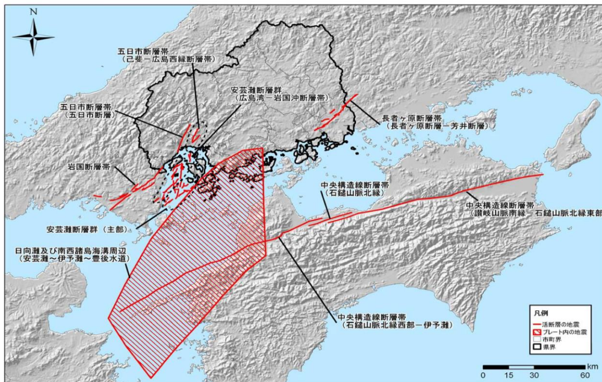
図 6 想定地震位置図（既に明らかとなっている断層等を震源とする地震）
