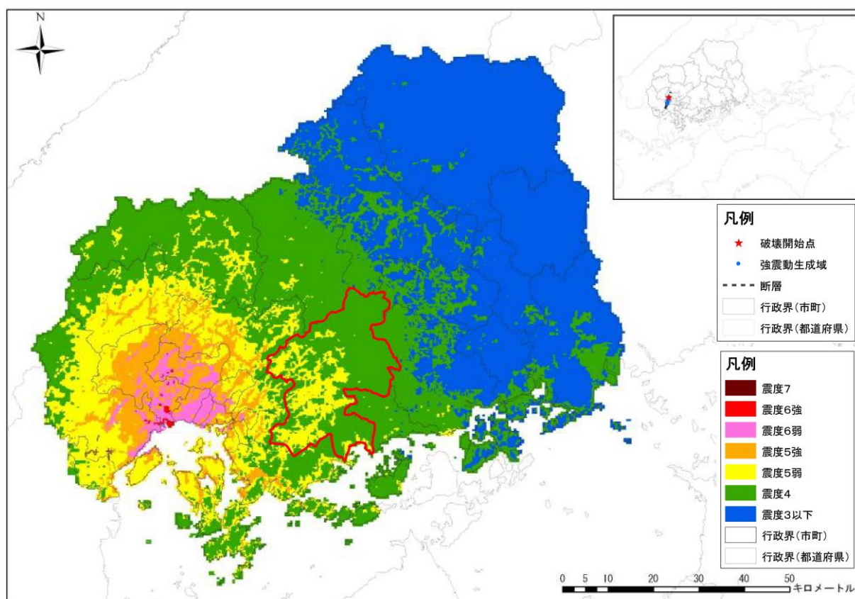
図 7-7 地震の震度分布（五日市断層の地震（北から破壊））
