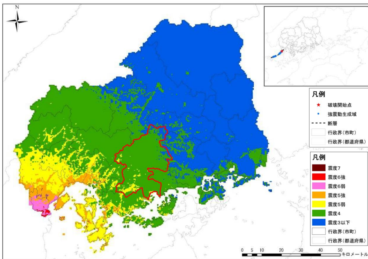
図 7-9 地震の震度分布（岩国断層帯の地震（東から破壊））
