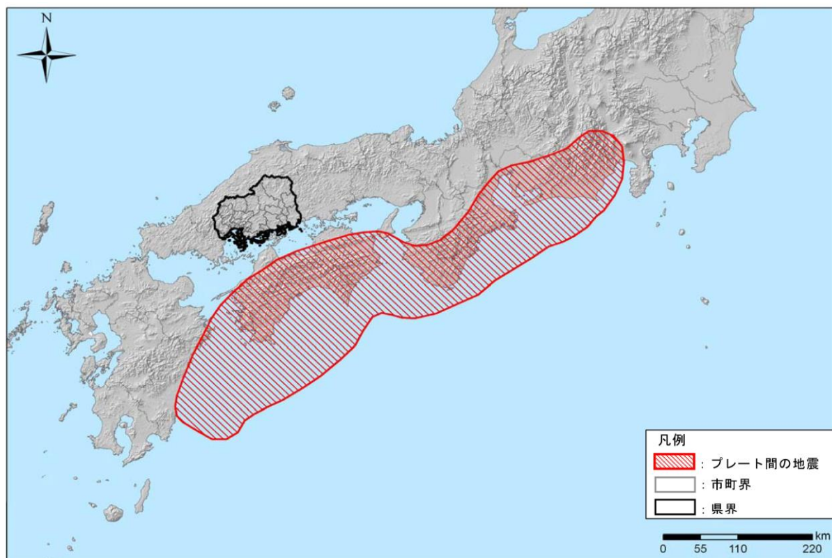
図 5 想定地震位置図（南海トラフ巨大地震）
