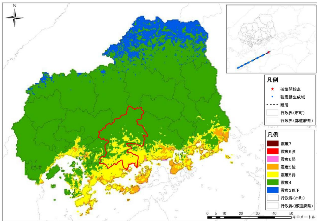
図 7-6 地震の震度分布（石鎚山脈北縁西部-伊予灘の地震（東から破壊））
