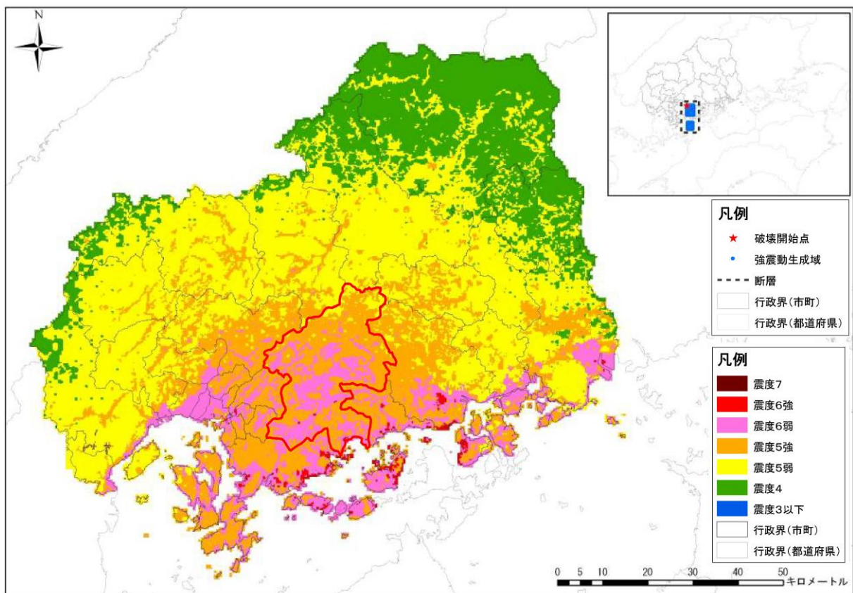
図 7-3 地震の震度分布（安芸灘～伊予灘～豊後水道の地震（北から破壊））
