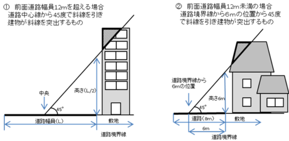
図 11 通行障害建築物の概要
