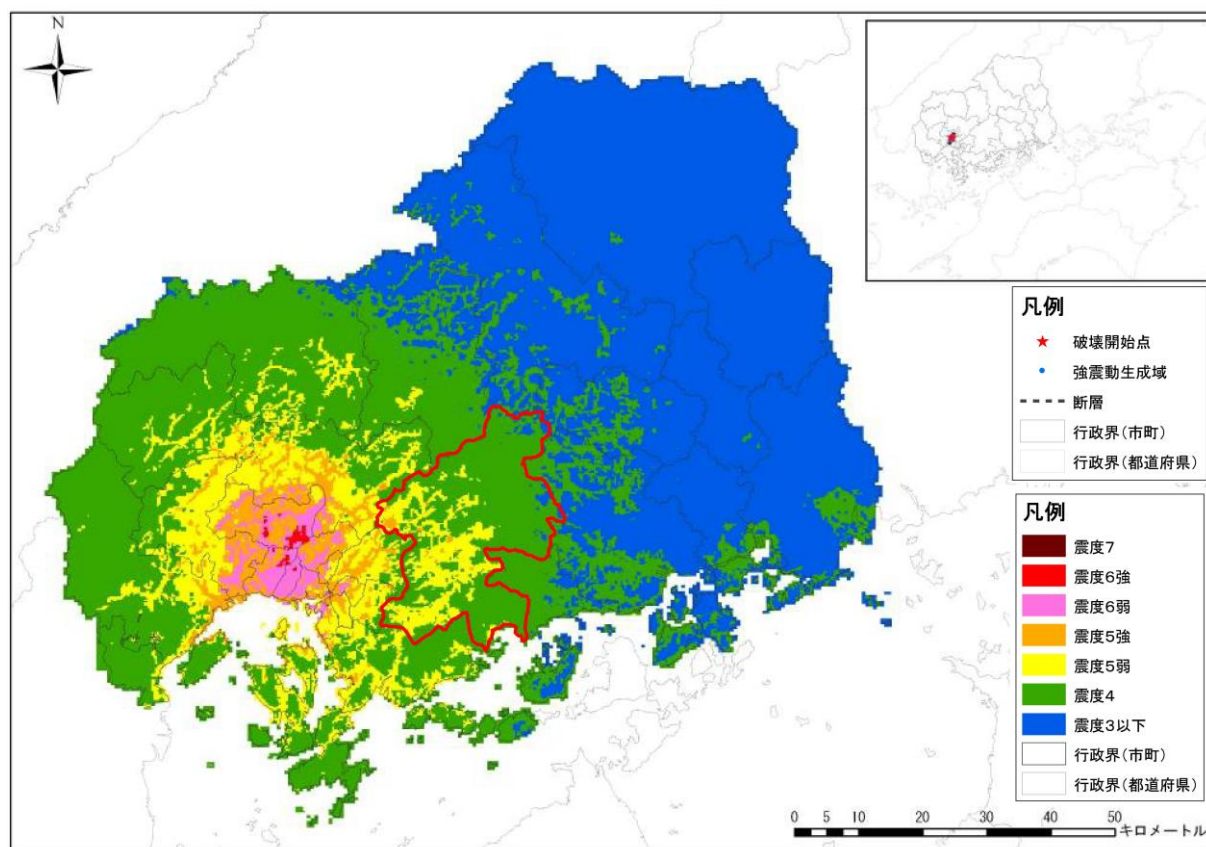
図 7-8 地震の震度分布（己斐-広島西縁断層帯の地震（M6.5）（北から破壊））
