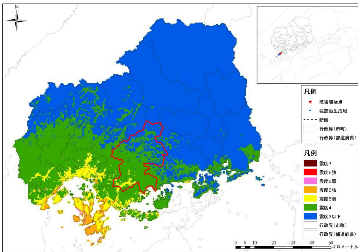
図 7-10 地震の震度分布（安芸灘断層群（主部）の地震（北から破壊））
