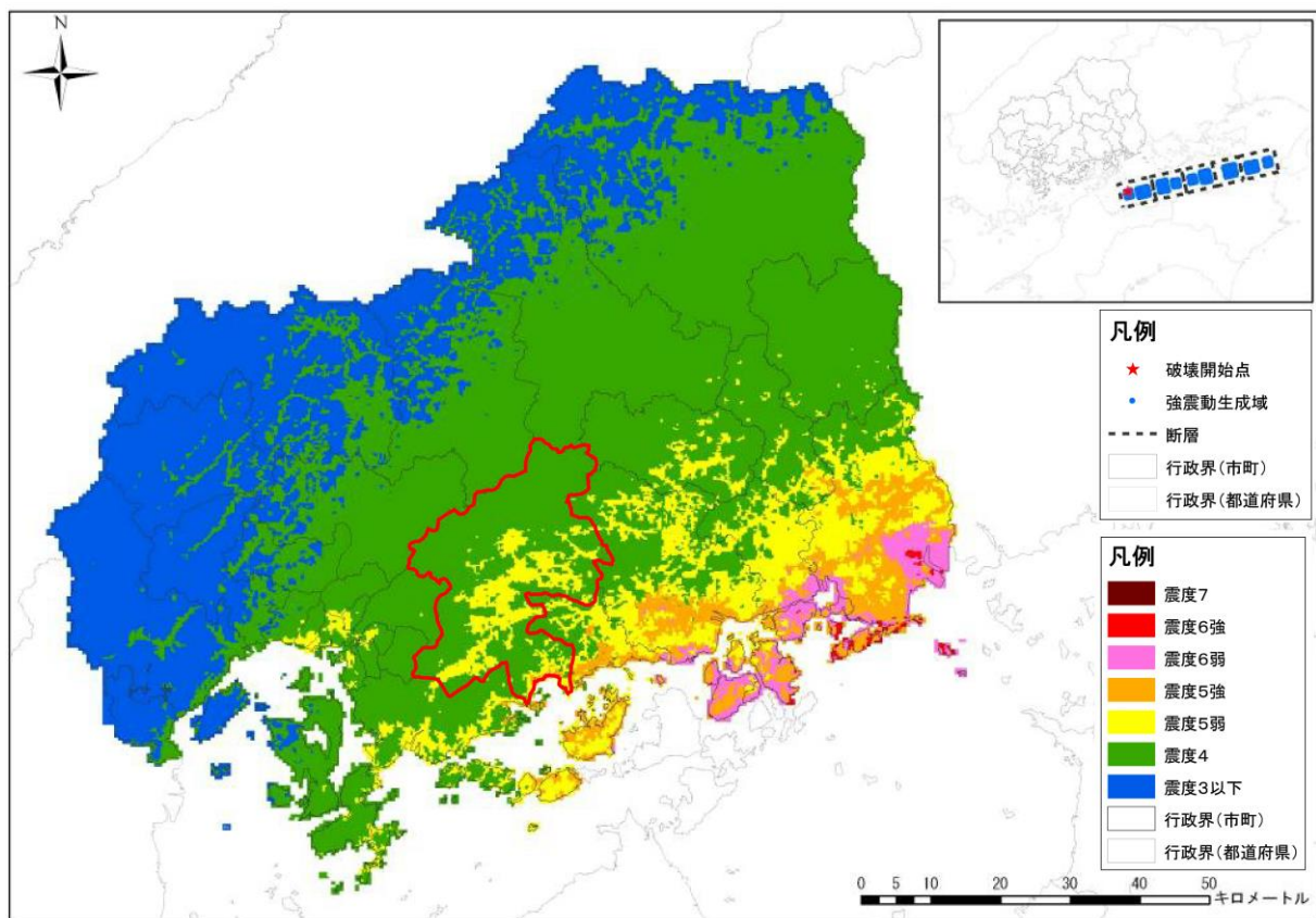
図 7-4 地震の震度分布（讃岐山脈南縁-石鎚山脈北縁東部の地震（西から破壊））
