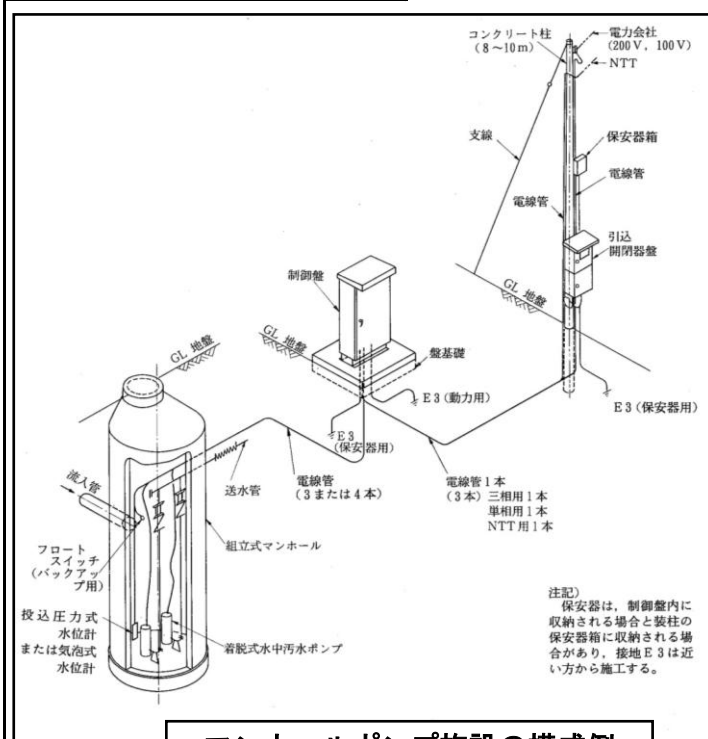
マンホールポンプ施設の構成例
