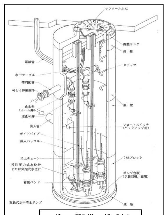
ポンプ設備の構成例
