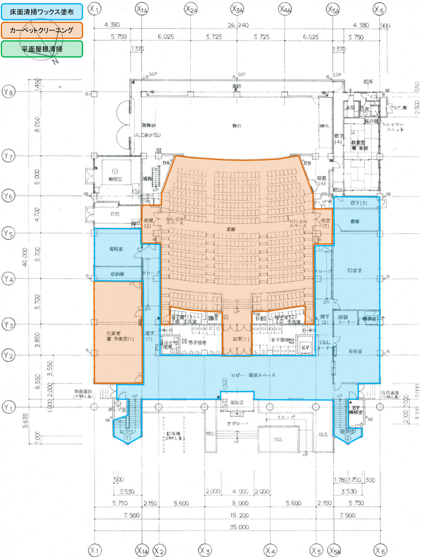
図1 平面図(1階)
