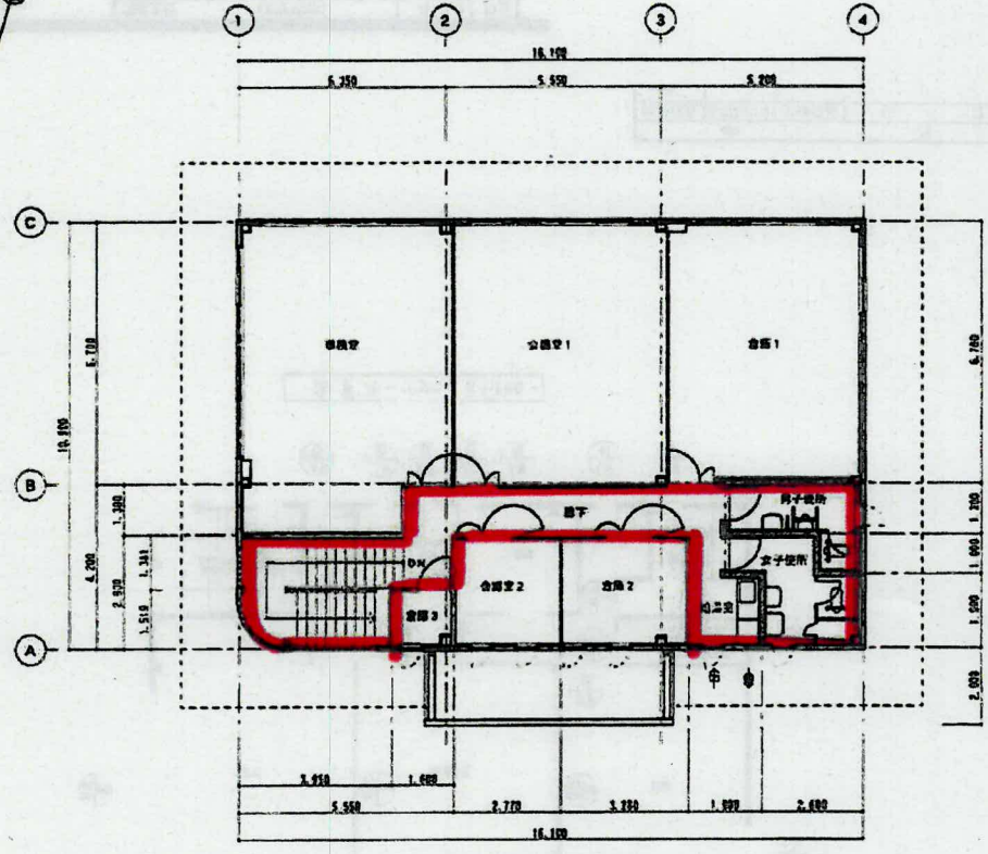
2階平面図 1/100
