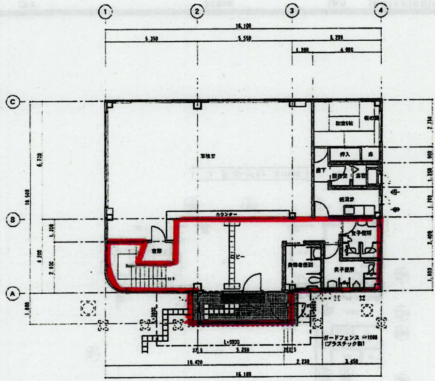
1階平面図 1/100
