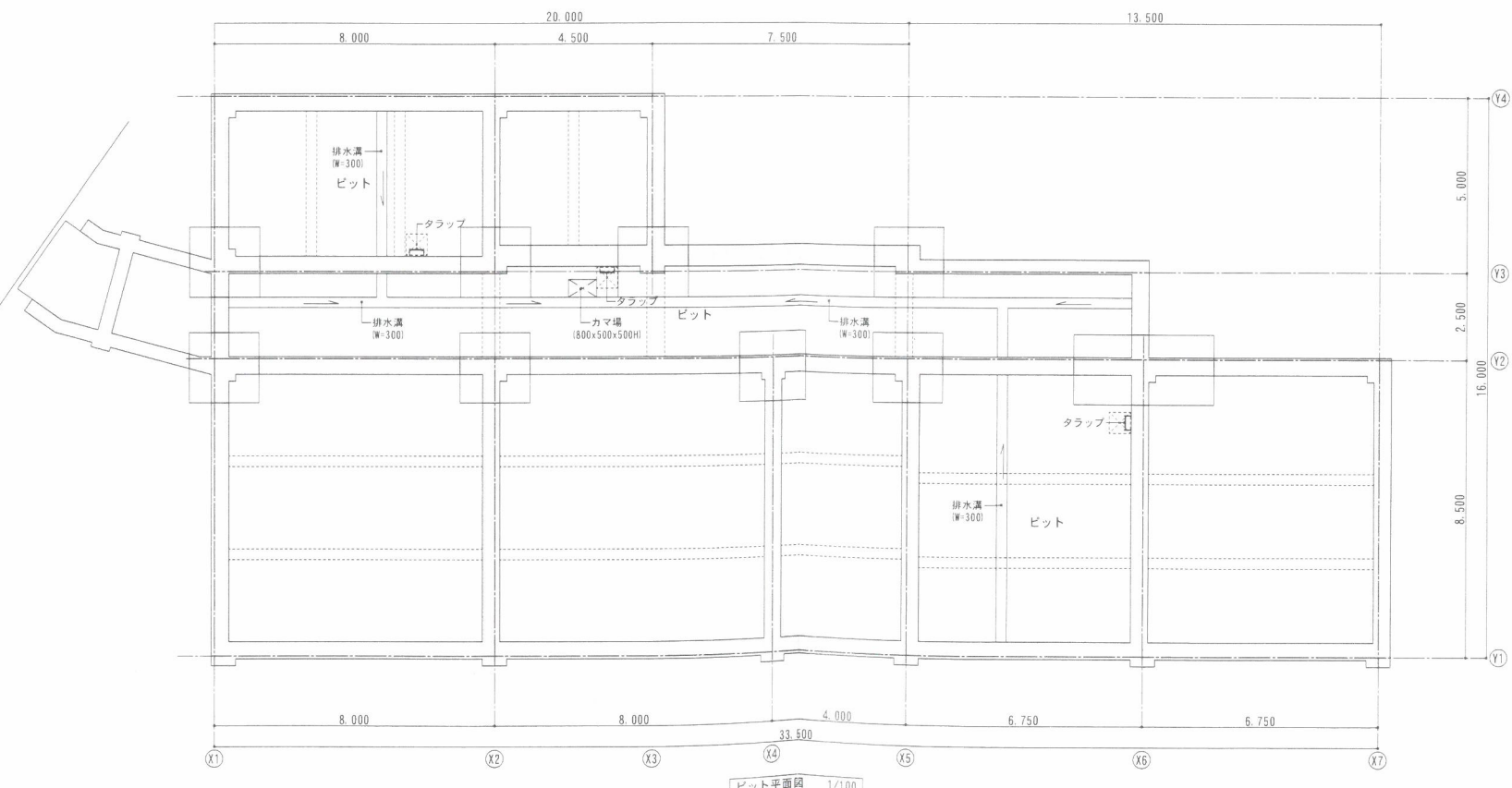
ピット平面図 1/100
