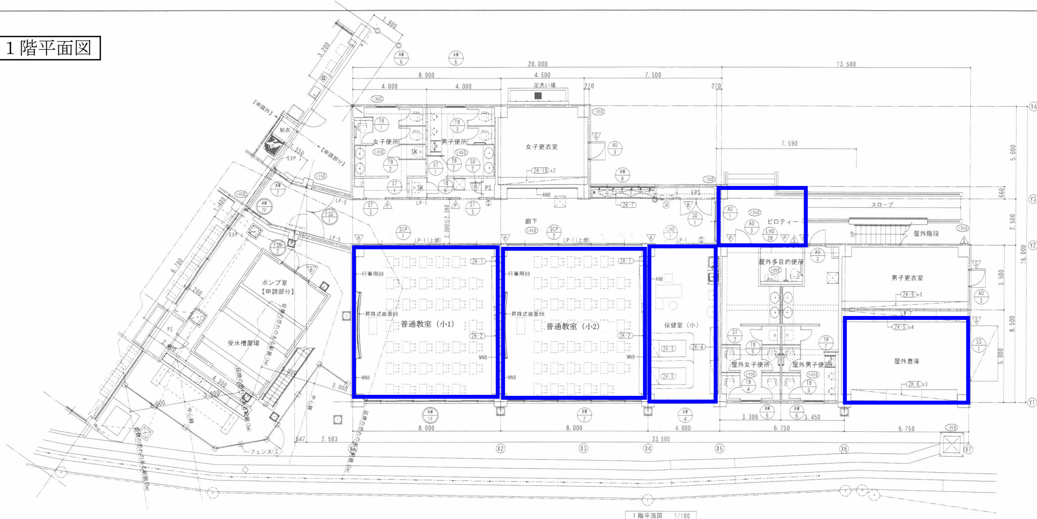
1階平面図 1/100
