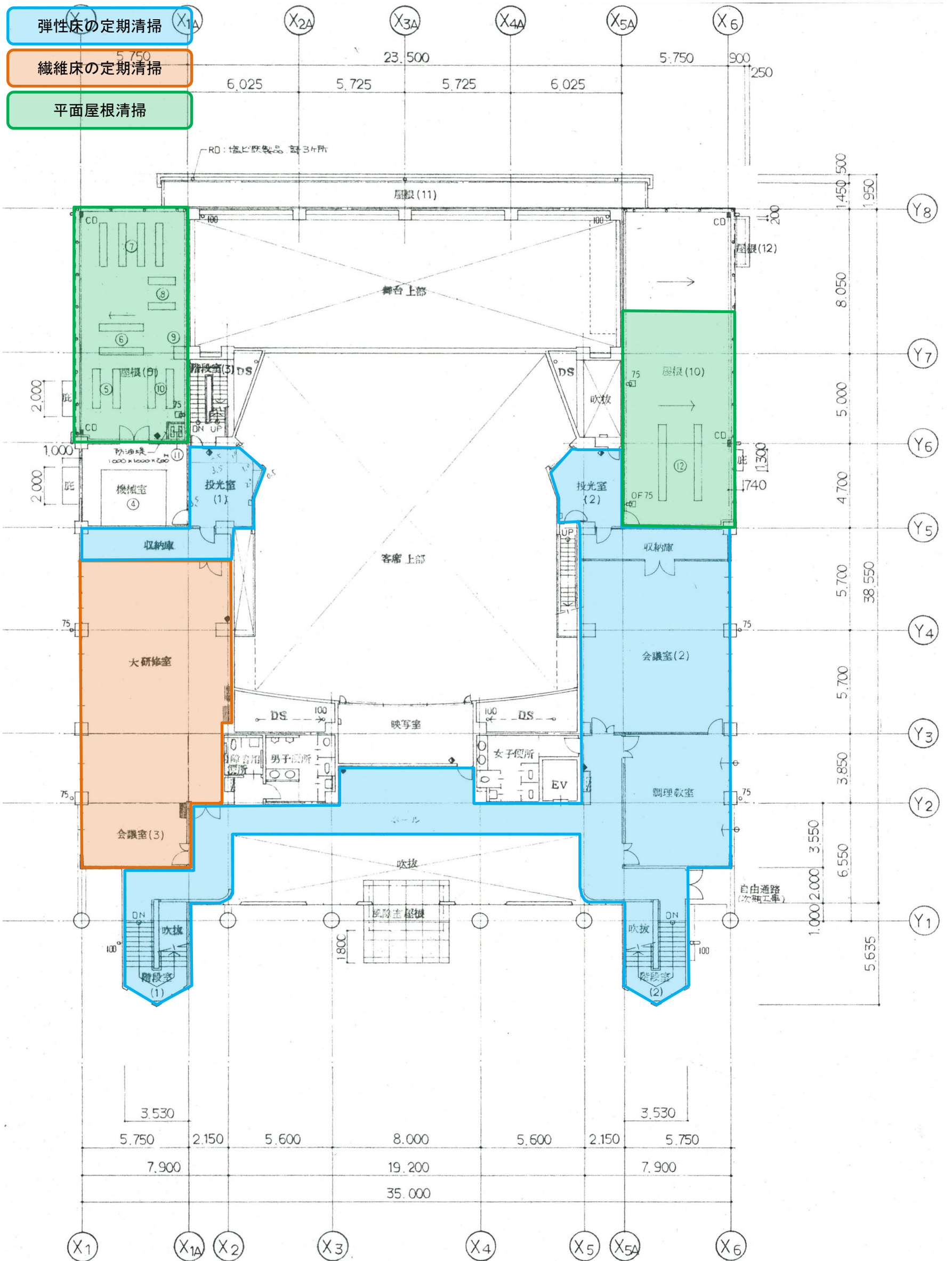
図2 豊栄生涯学習センター平面図(2階)
