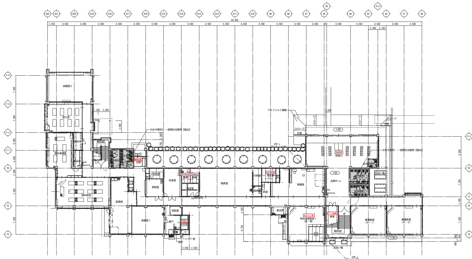
1階平面図 (既設校舎) S=1/200 ※改修内容については別図参照の事。
