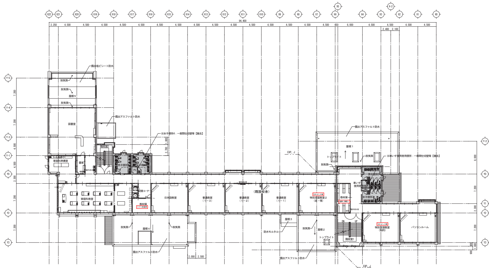
2階平面図 (既設校舎) S=1/200 ※改修内容については別図参照の事。
