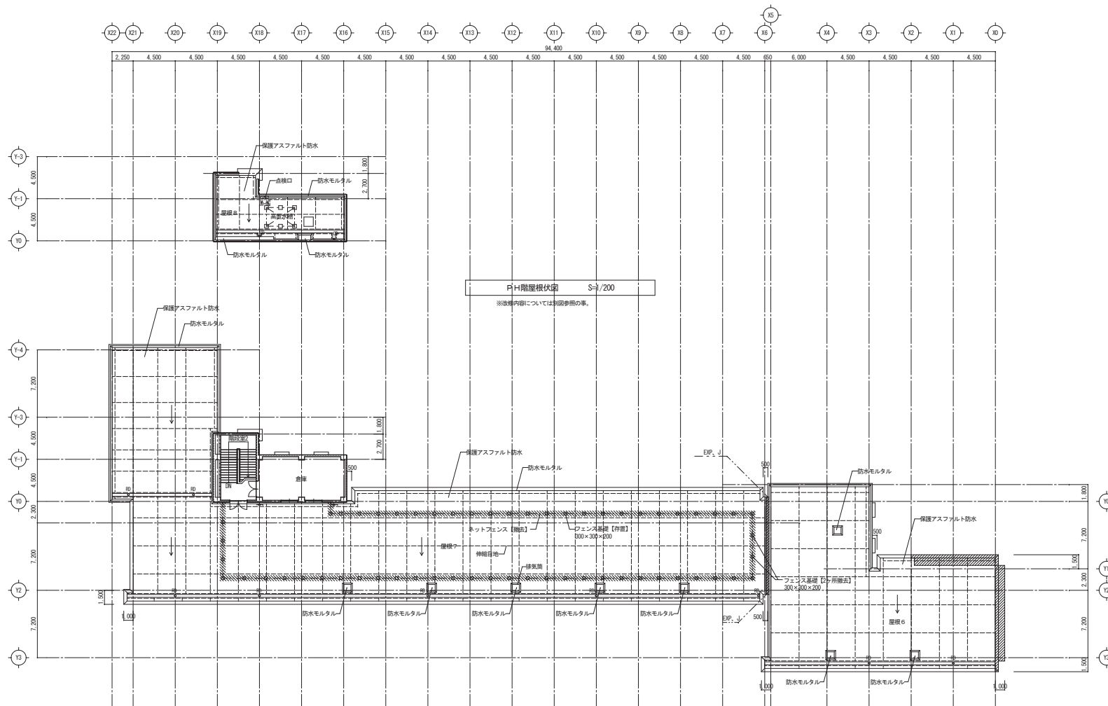
5階屋根伏図（既設校舎） S=1/200
