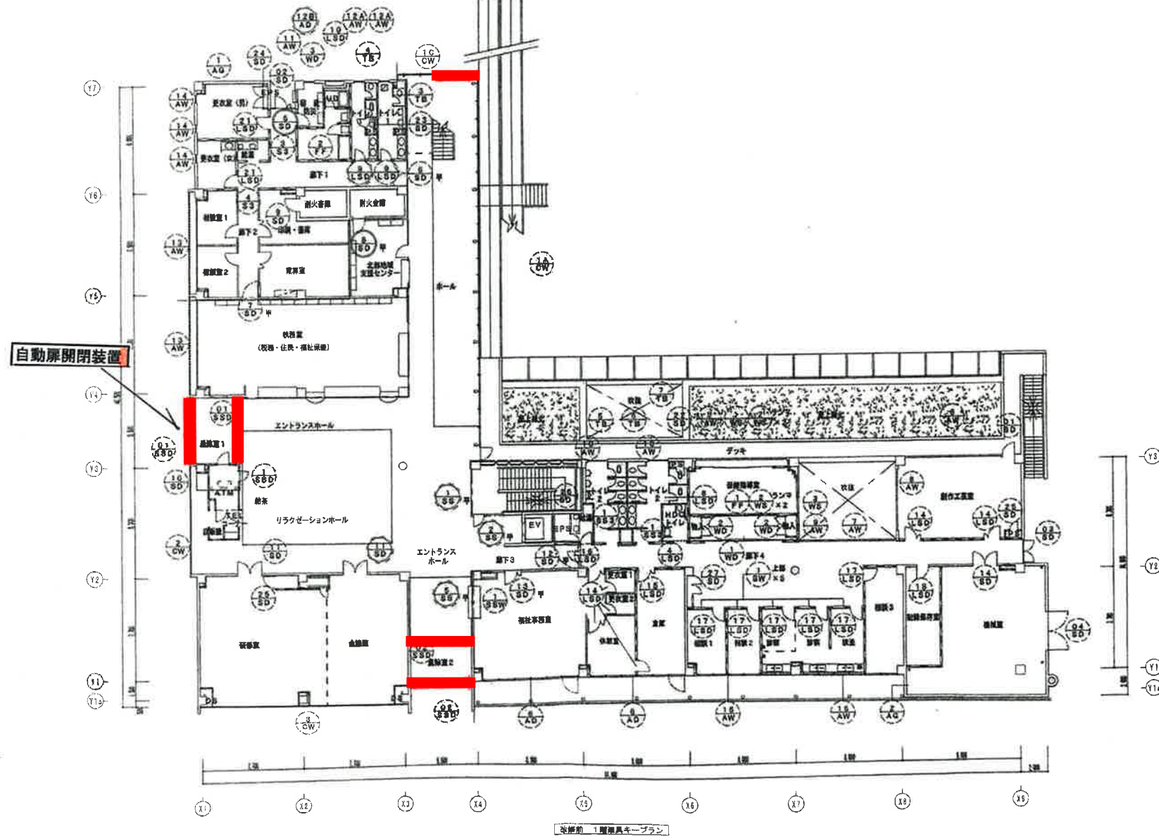
延焼前 1階器具キープラン
