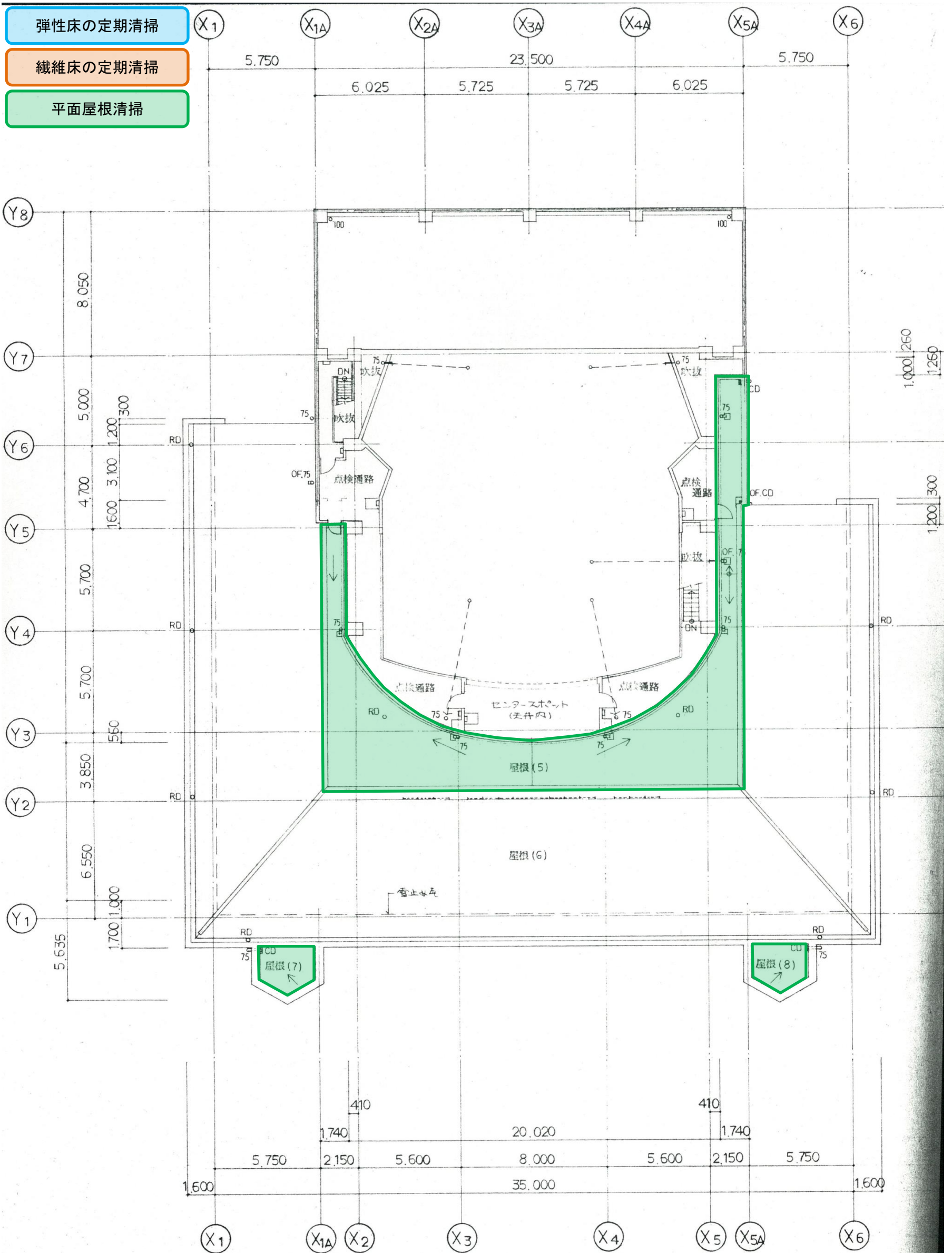
図3 豊栄生涯学習センター平面図(屋根裏)
