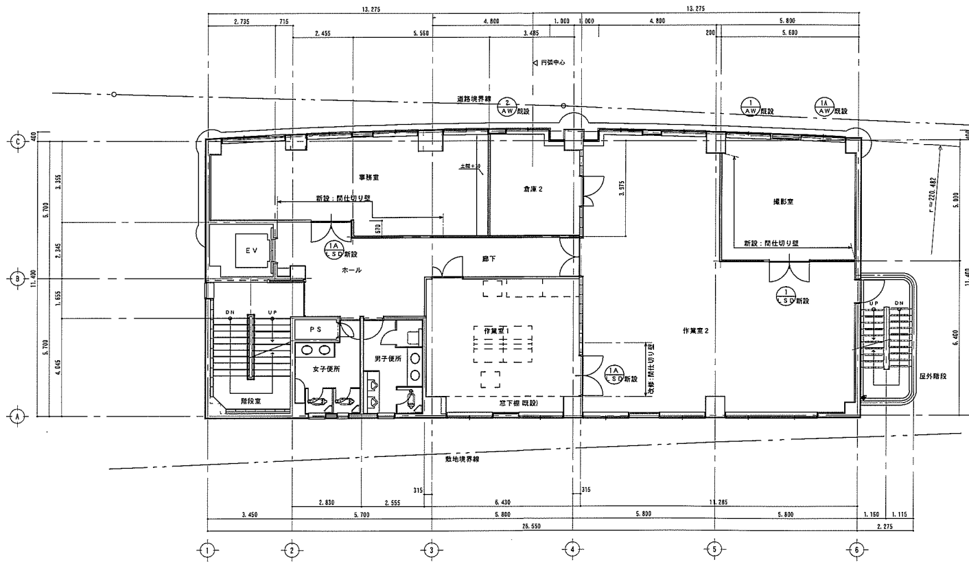
東広島市出土文化財管理センター3階平面図
