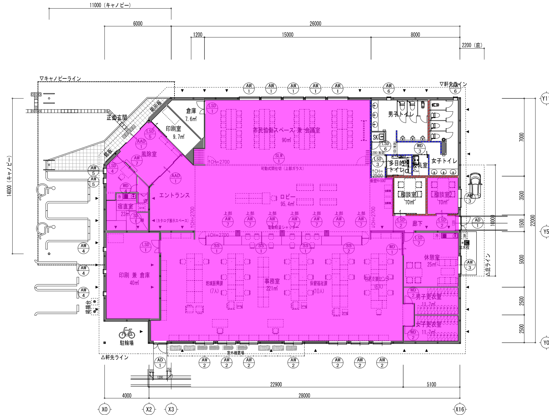
平面図 S=1/200
