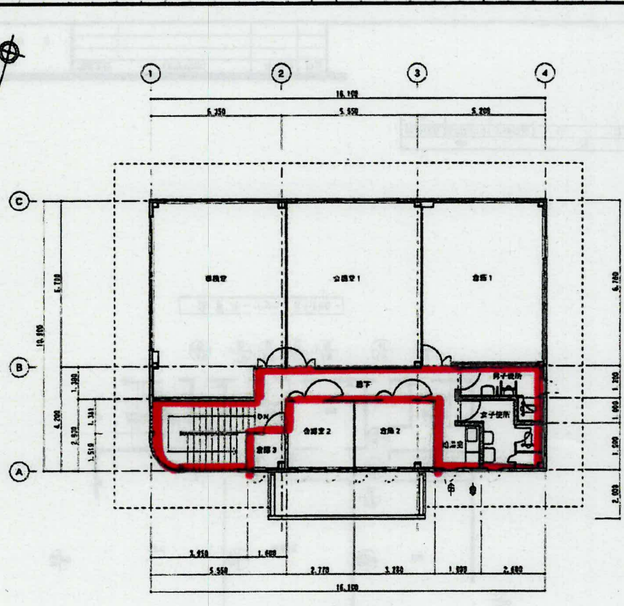
2階平面図 1/100
