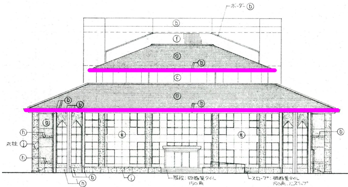
北立面図
