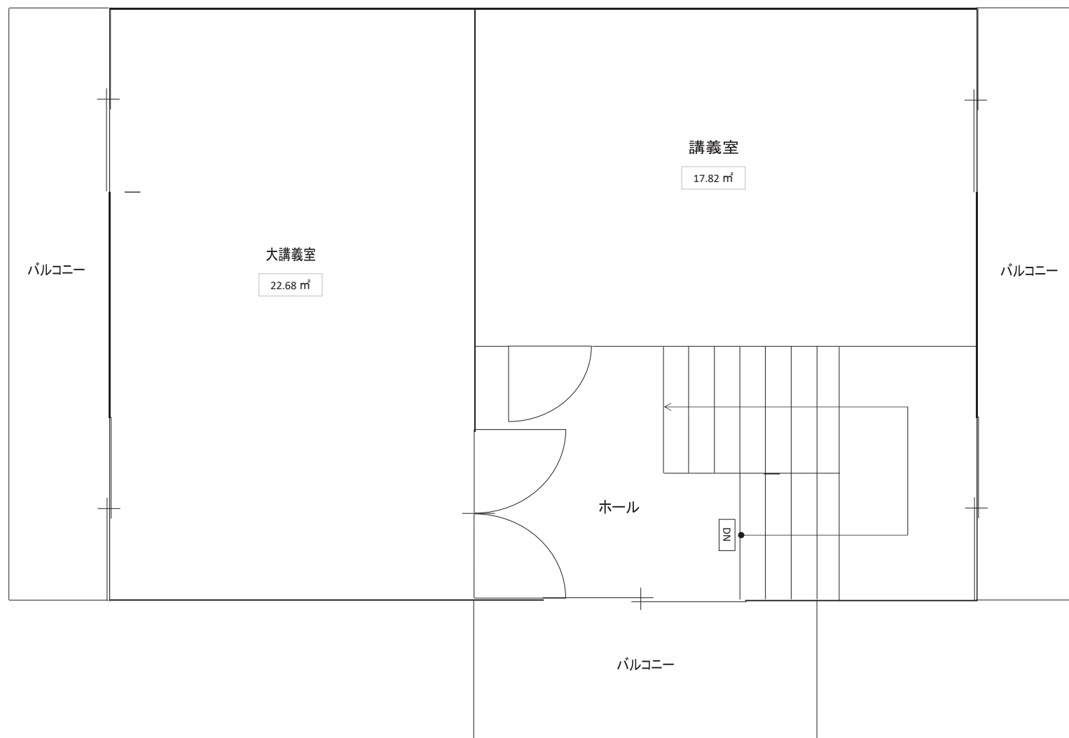
安芸津人権センター（旧教育・2F）
