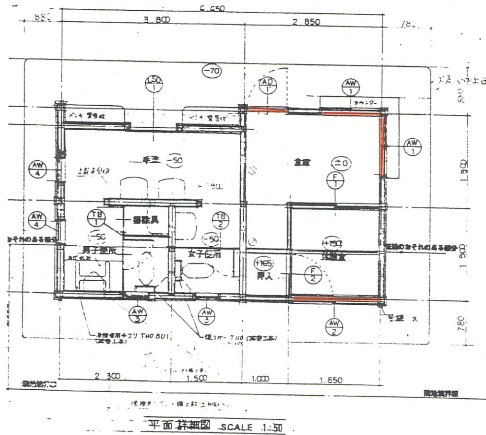
東広島市指定重要文化財旧石井家住宅管理棟平面図
