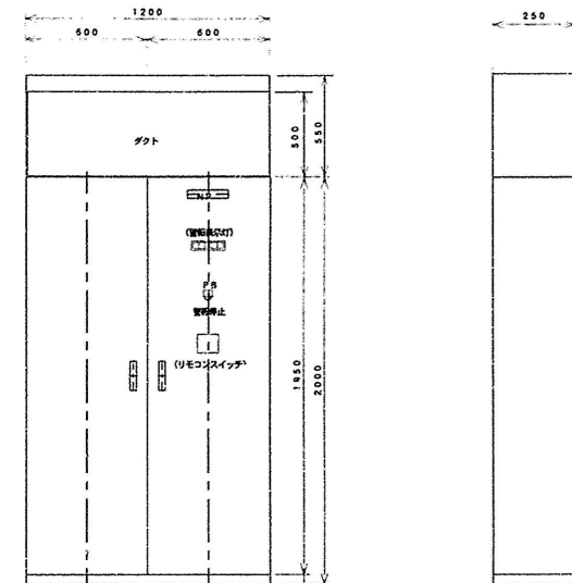
電圧分電盤 (PL-1) 単体図 1/20
