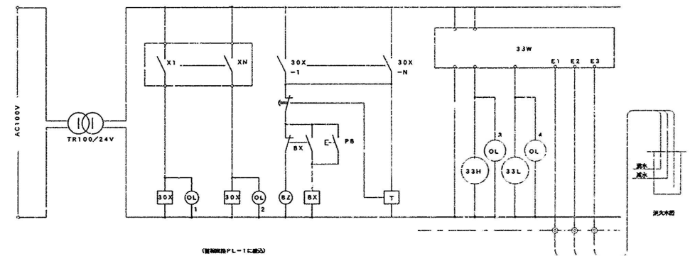
電圧分電盤 (PL-1) 単体図 1/20
