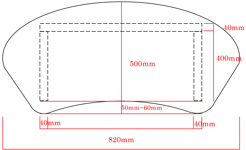
設計図 4 カウンター
