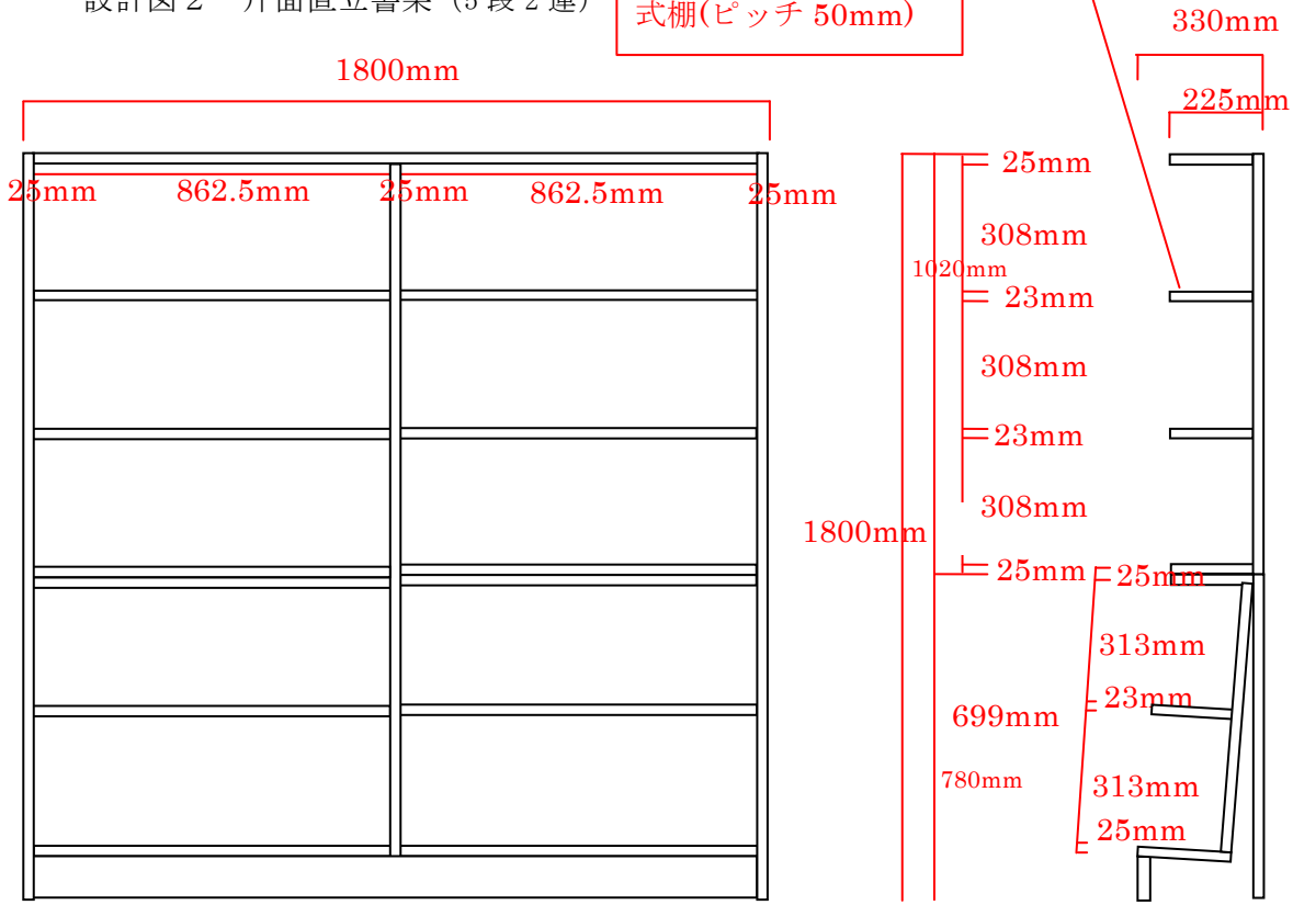
設計図 2 片面直立書架 (5段2連)
