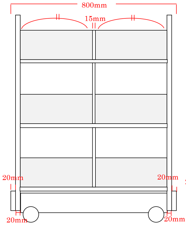
設計図 3 ブックトラック
