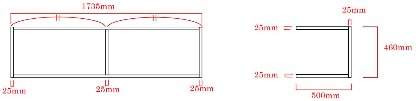
設計図 6 本棚 B
