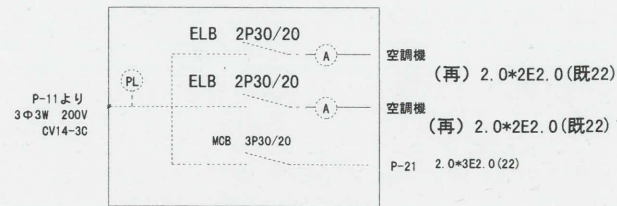
既設 P-B改修結線図
