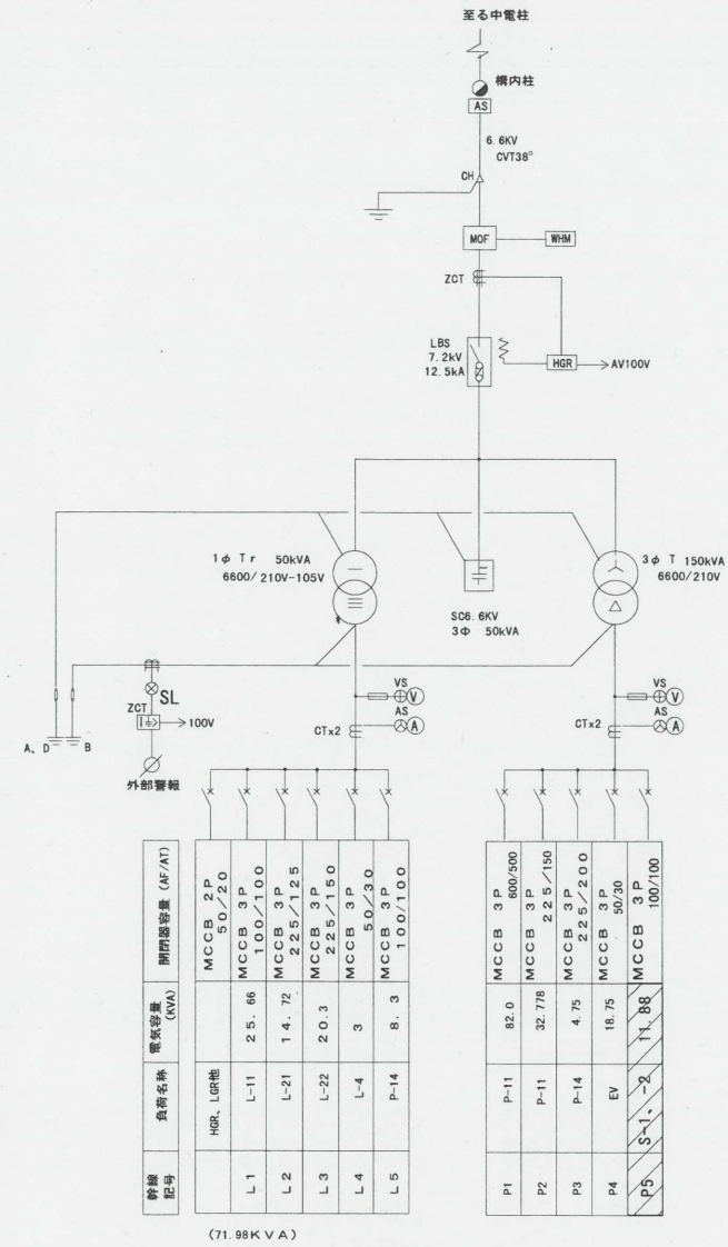
受変電設備結線図
