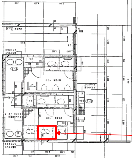
便所詳細
