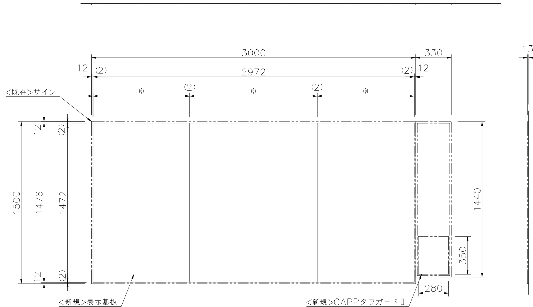
外観図
