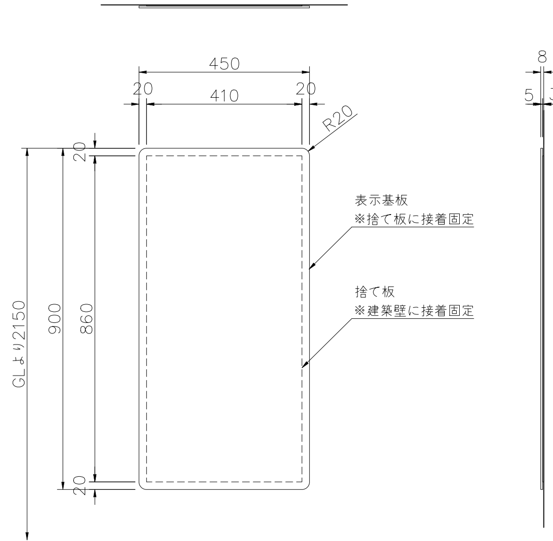
外観図
