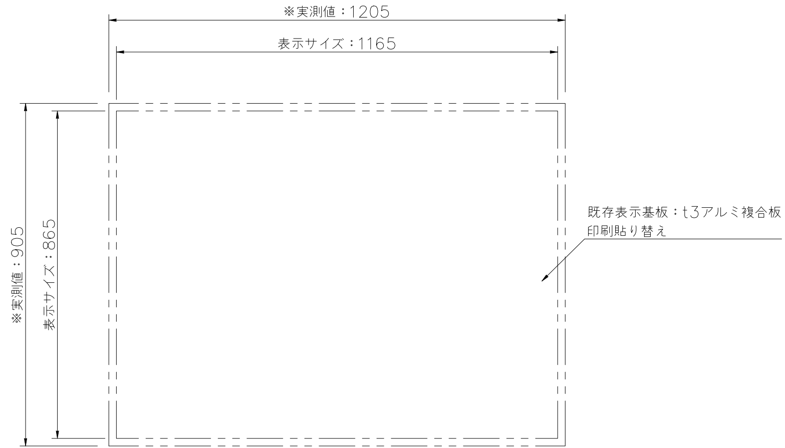
外観図
