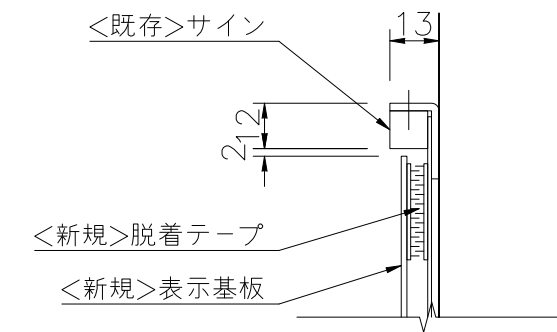
断面詳細図
