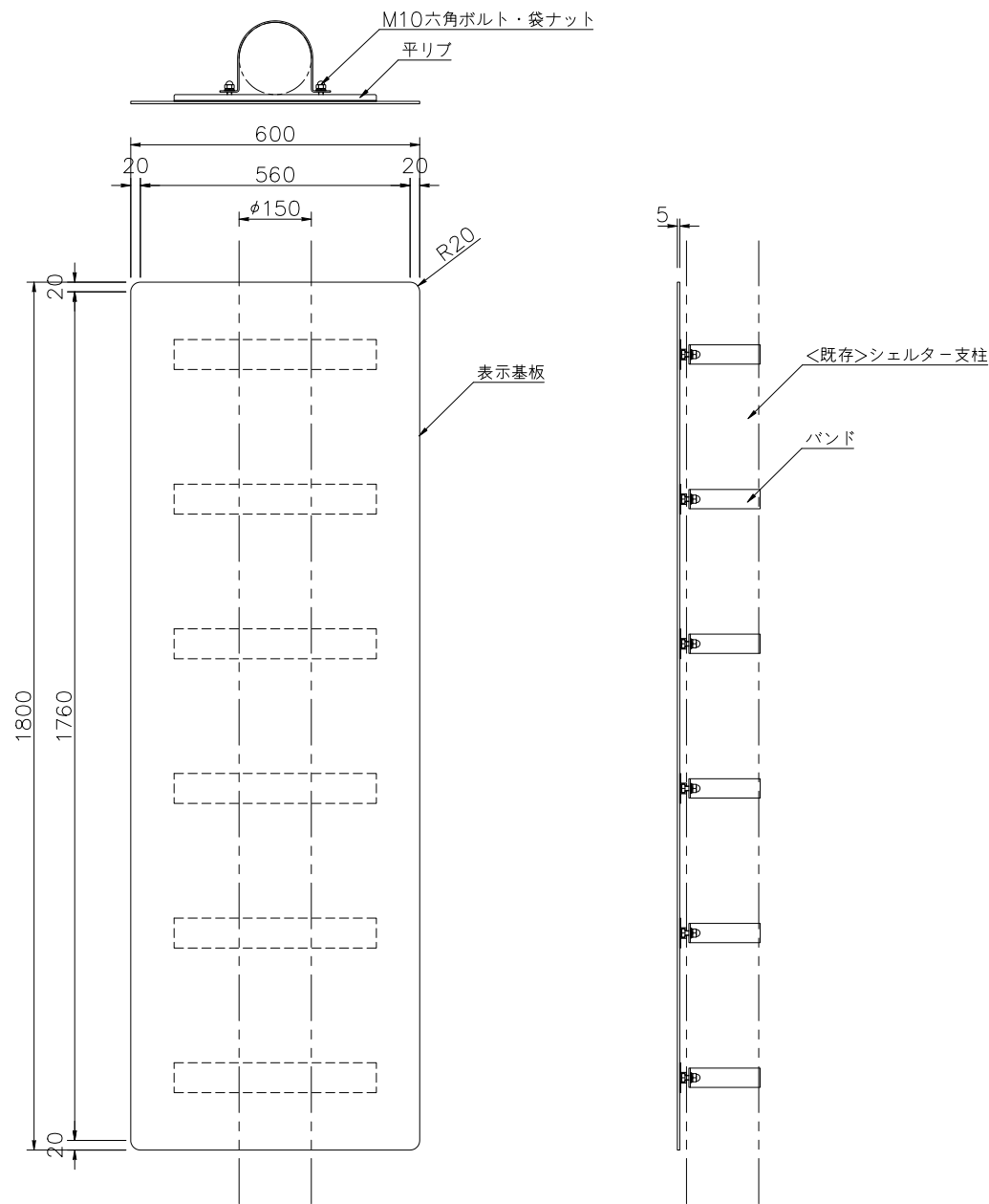
外観図
