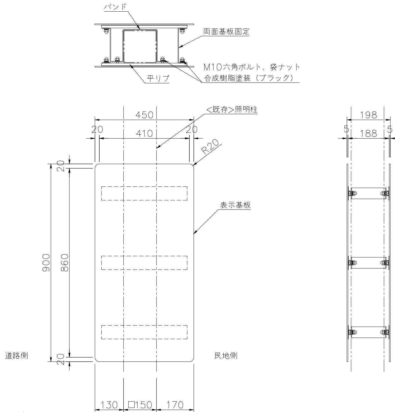
外観図
