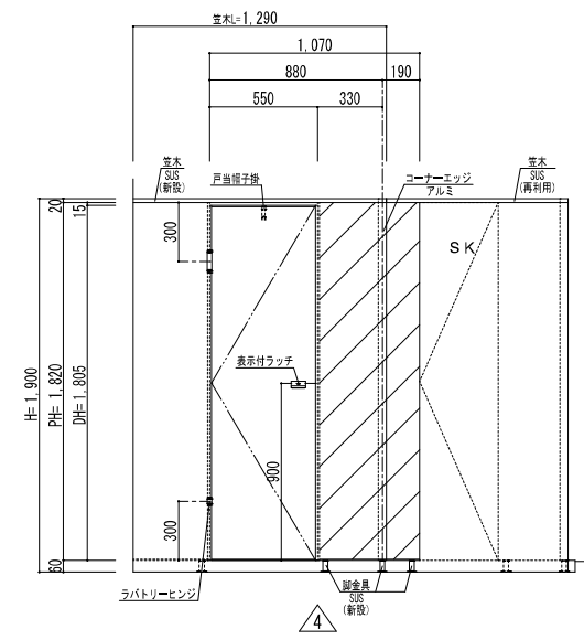
展開図
