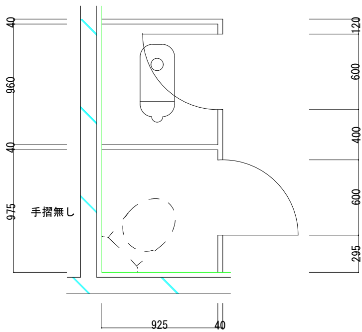
女子トイレ 1/30
