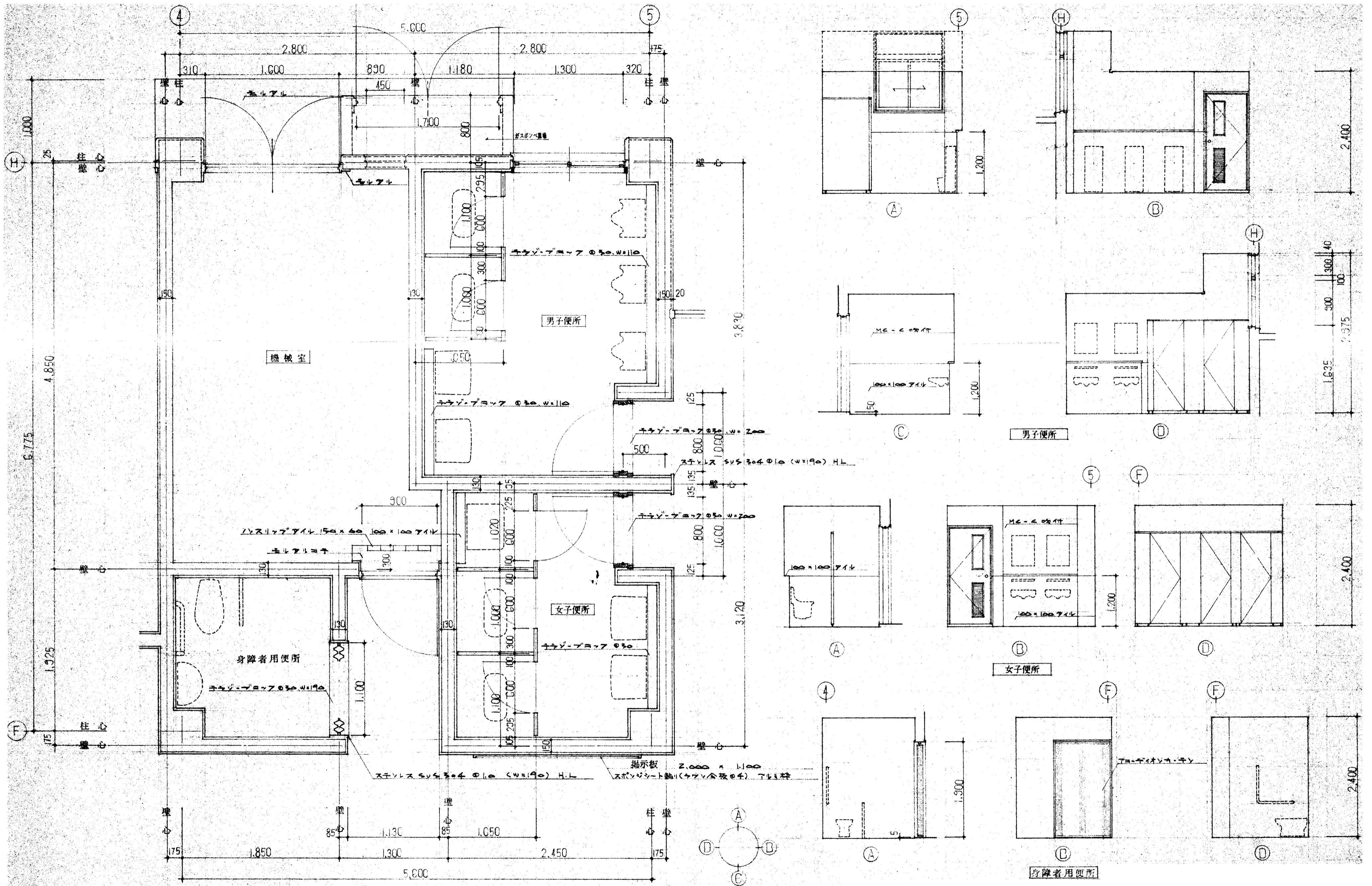
平面詳細図 1:30
