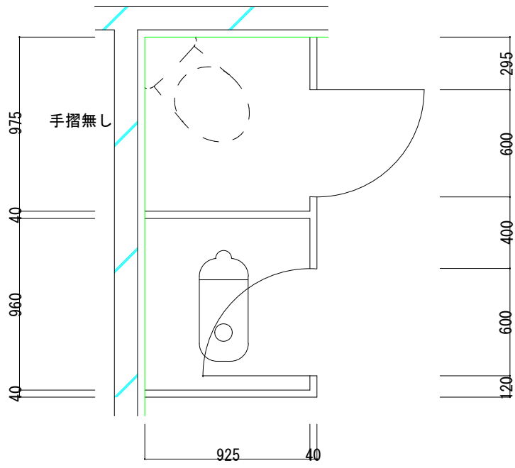
男子トイレ 1/30
