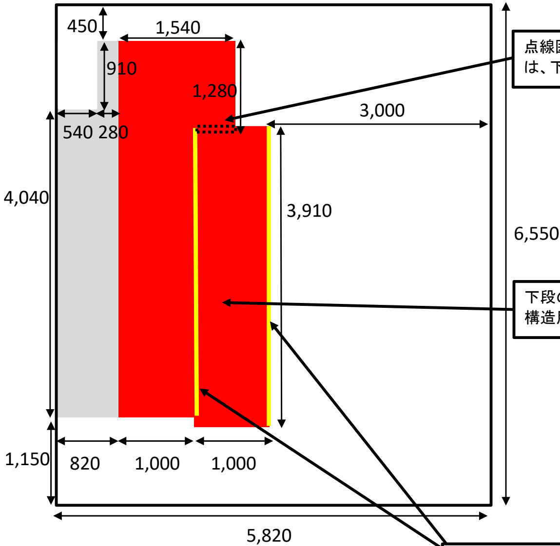
屋上西側 平面図
