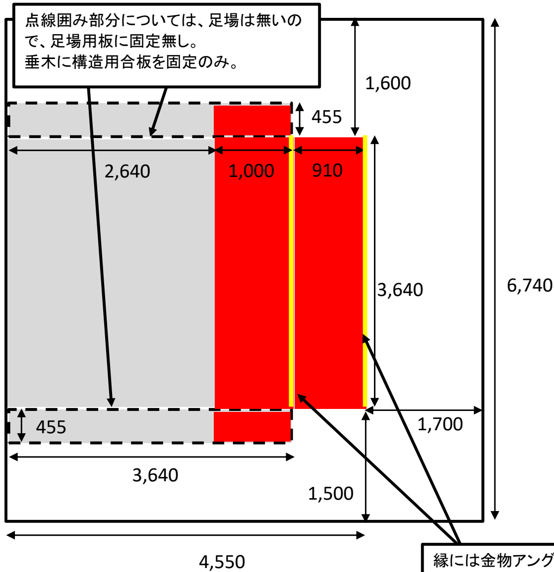
屋上東側 平面図
