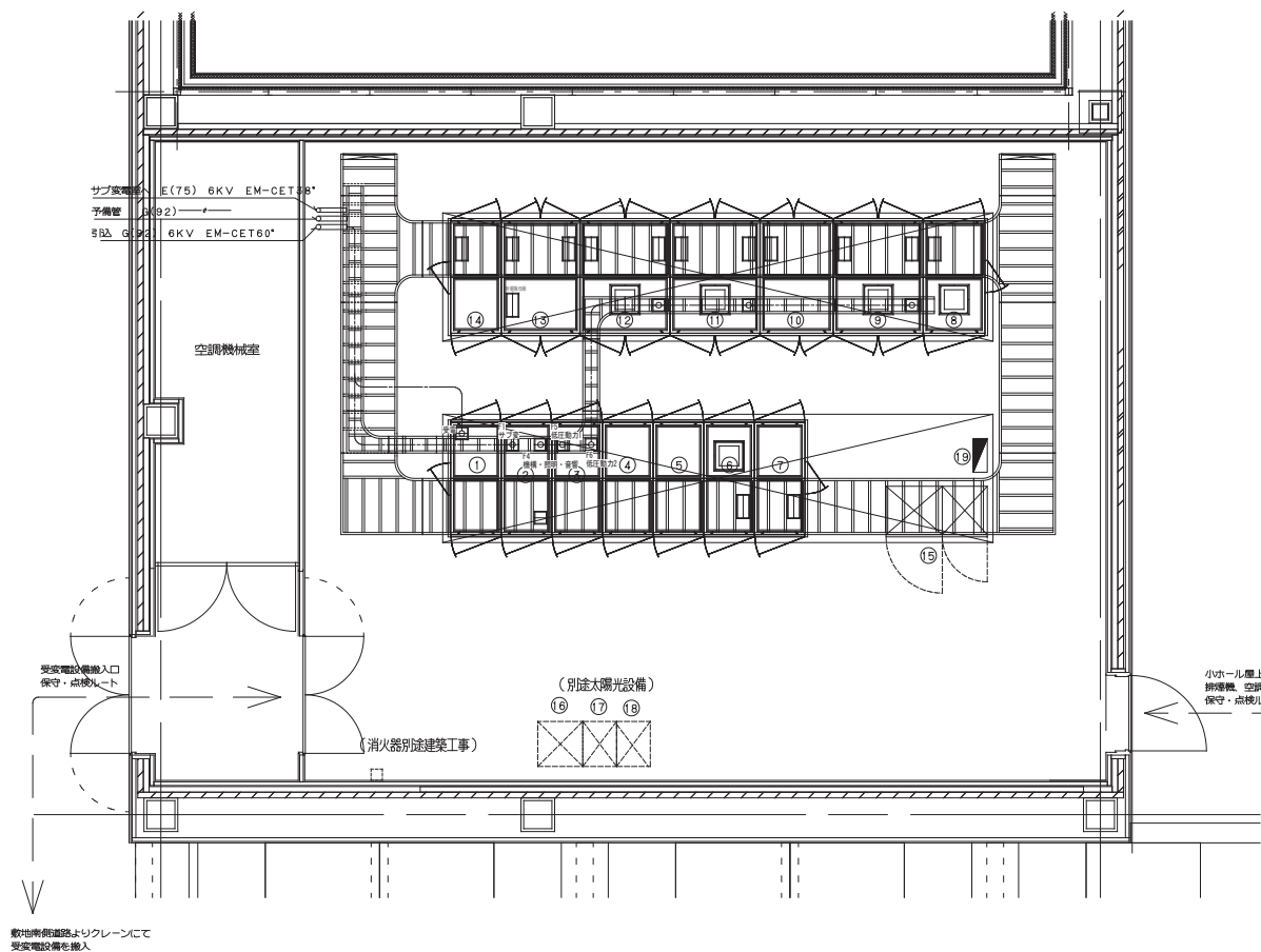
電気室 配置図
