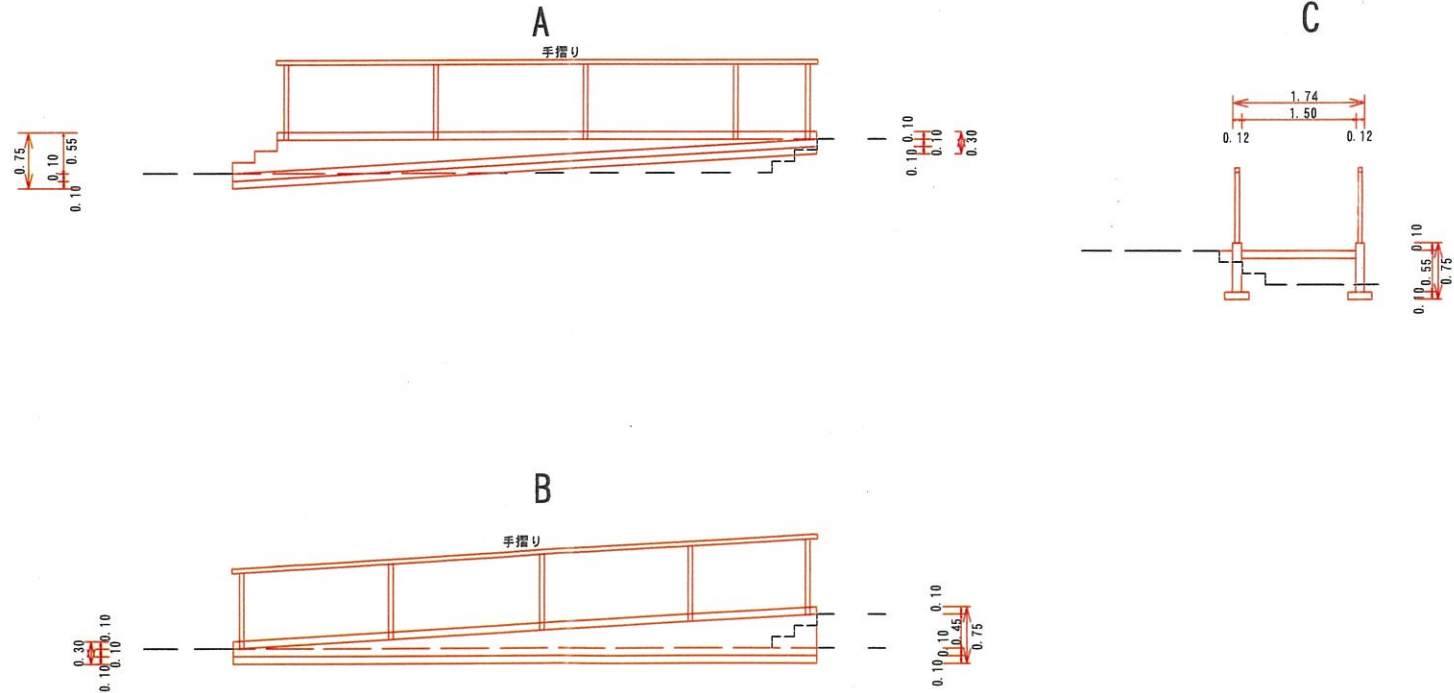
断面図
