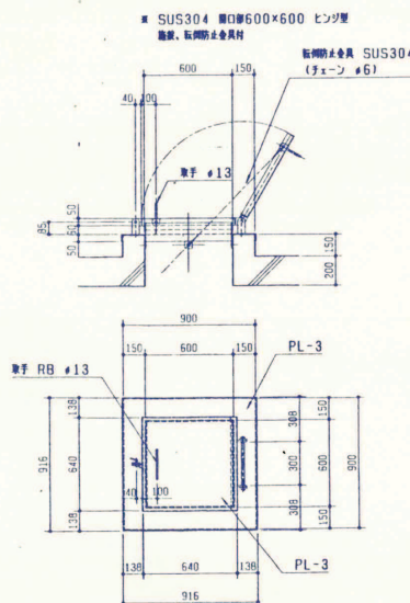
人孔蓋詳細図
