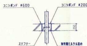
a詳細図
