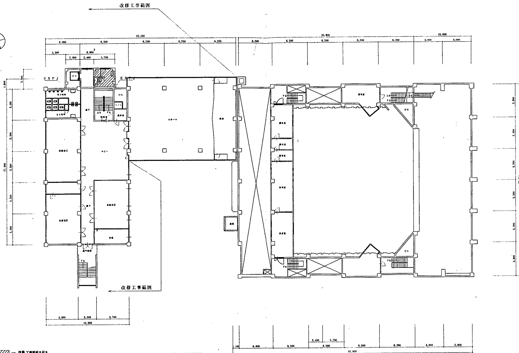
3階平面図 1:200
