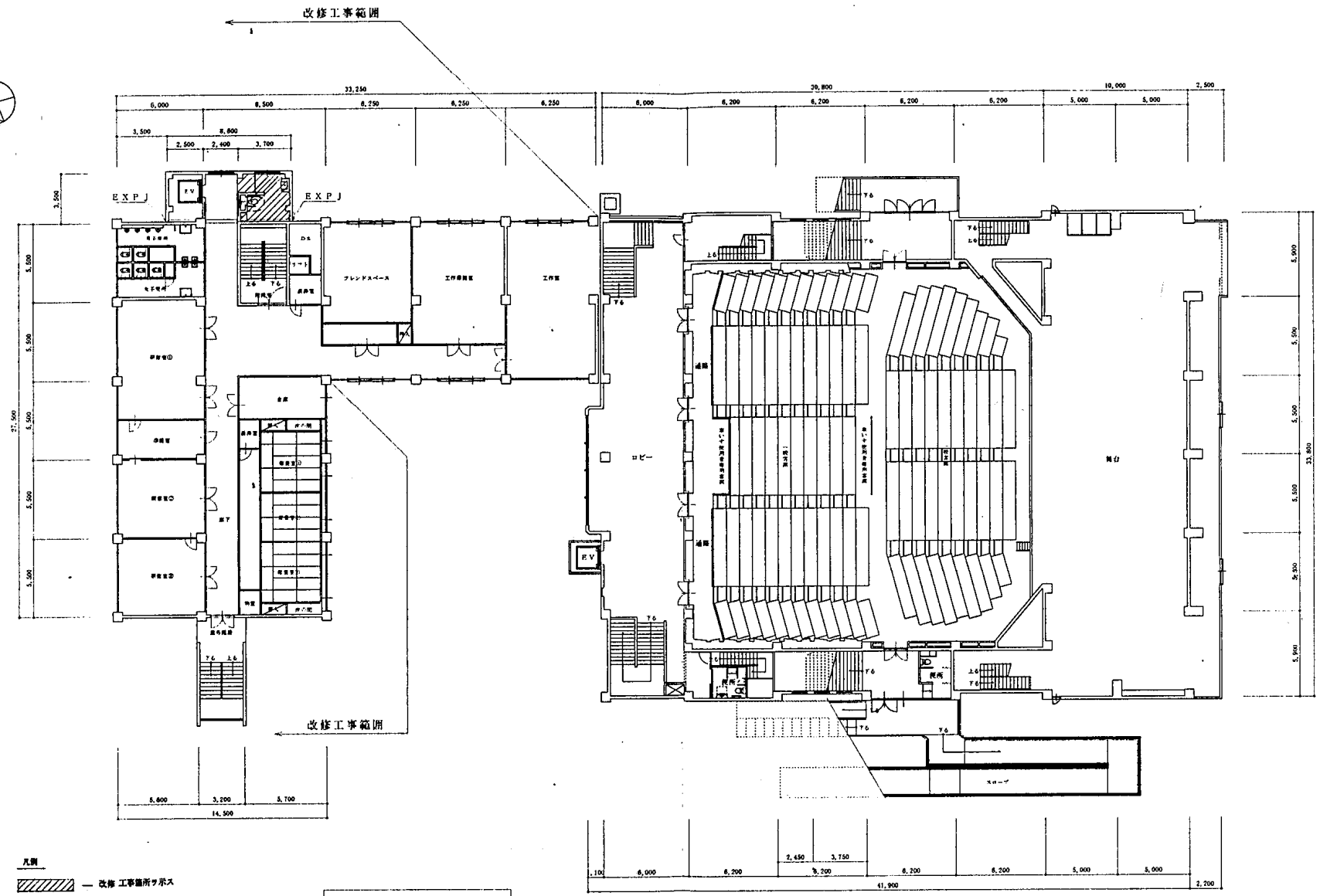
2階平面図 1 : 200
