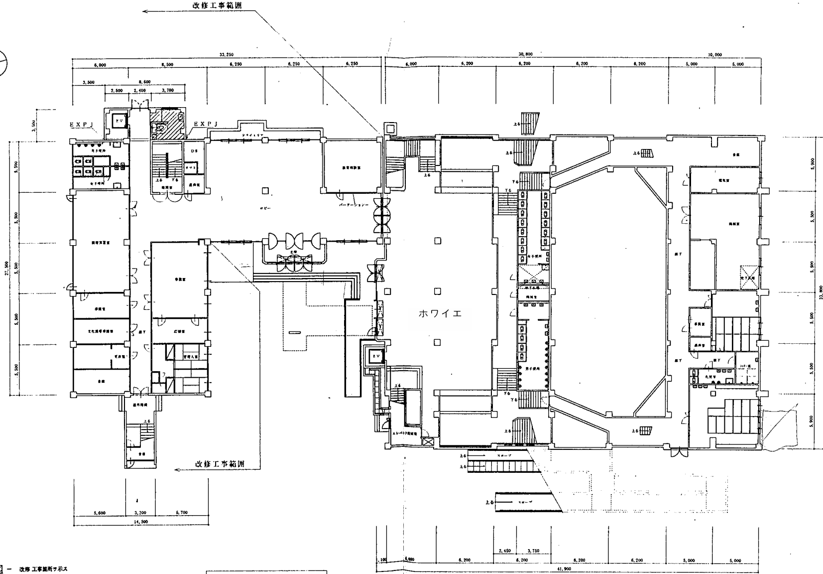
1階平面図 1:200
