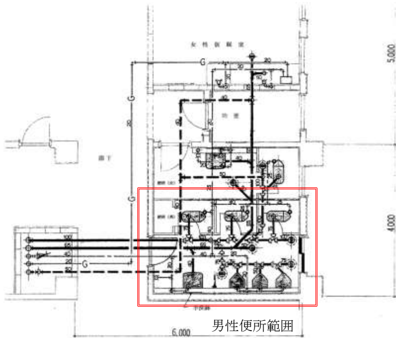
2階平面図(配管図)
