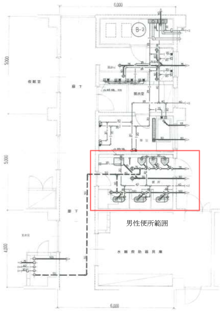
1 階 平 面 図 ( 配 管 図 )
