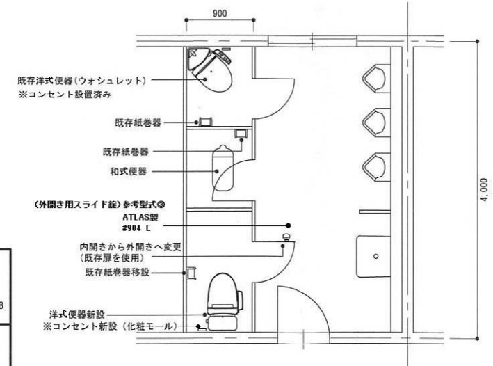
修繕 2階男子便所平面図 S=1/50
