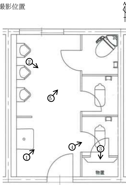
1階図面
