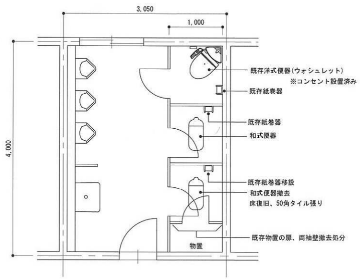
既存 1階男子便所平面図 S=1/50
