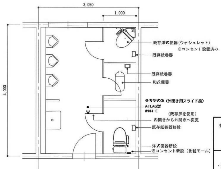
修繕 1階男子便所平面図 S=1/50
