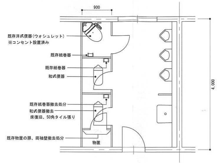
既存 2階男子便所平面図 S=1/50
