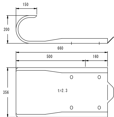
巻袖レール S=1/10
