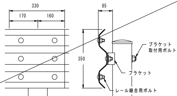
レール継合詳細
