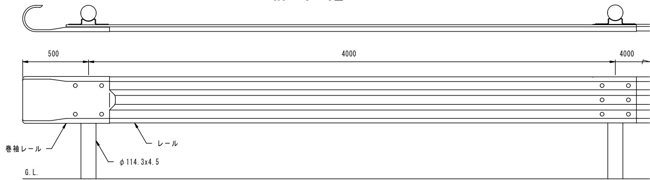
正面図
