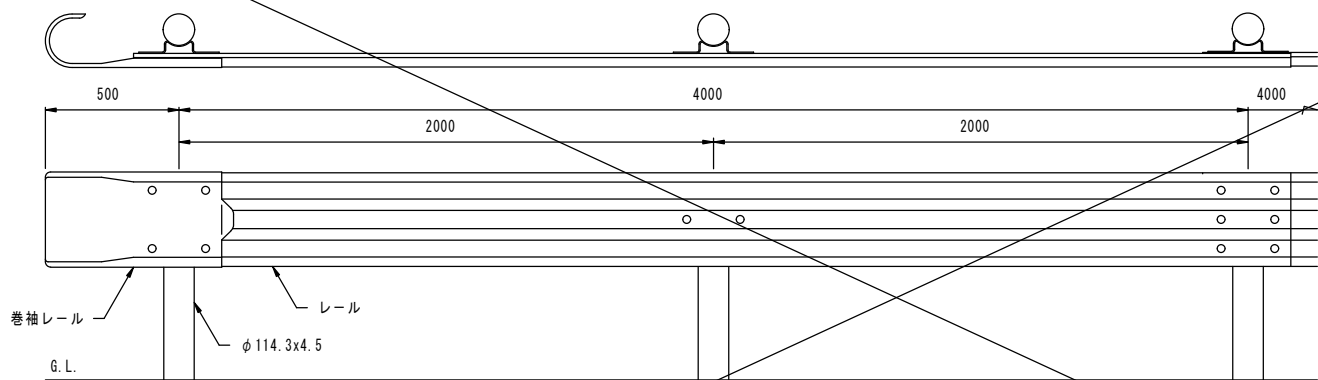
正面図
