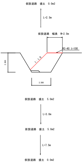
仮設道路 断面図
