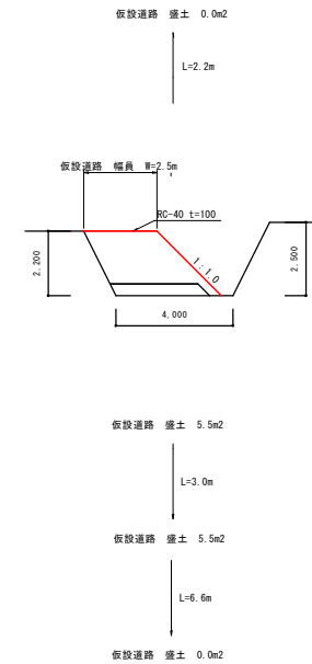
仮設道路 断面図
