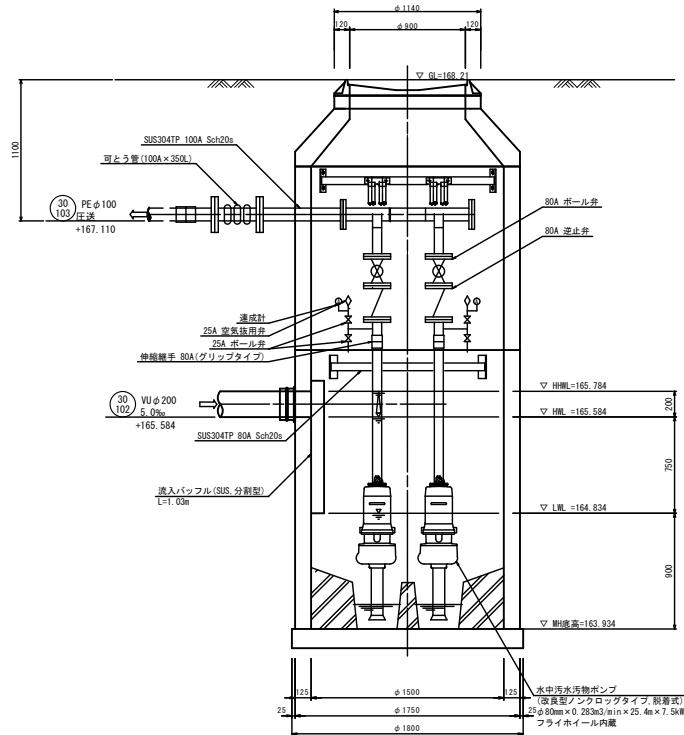
A-A断面図
