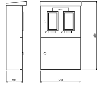
引込開閉器盤 S=1/10
