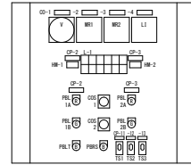
内部パネル図 S=1/10
