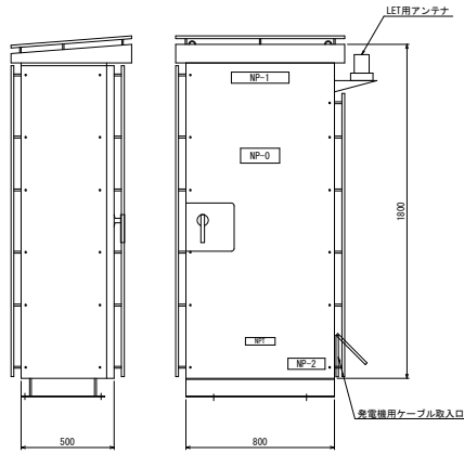
マンホールポンプ制御盤 S=1/15
