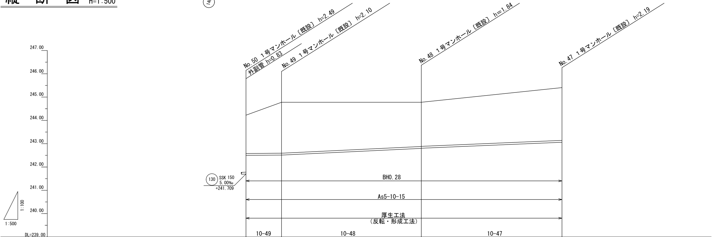
縦断面図 V=1:100 H=1:500
