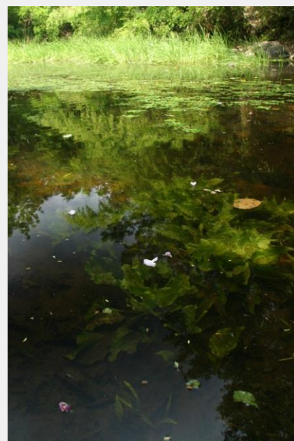
写真 3-7 ため池の水草
