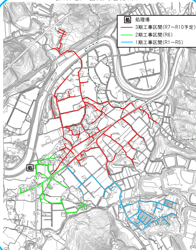
板城地区管路布設状況
